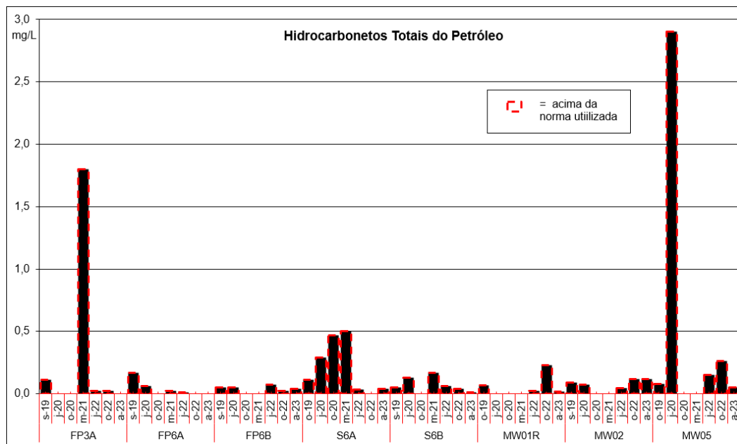
Figura 4.3 – Concentração em HTP na água de piezómetros localizados dentro e fora do Site 3001, entre 2019 e 2023
