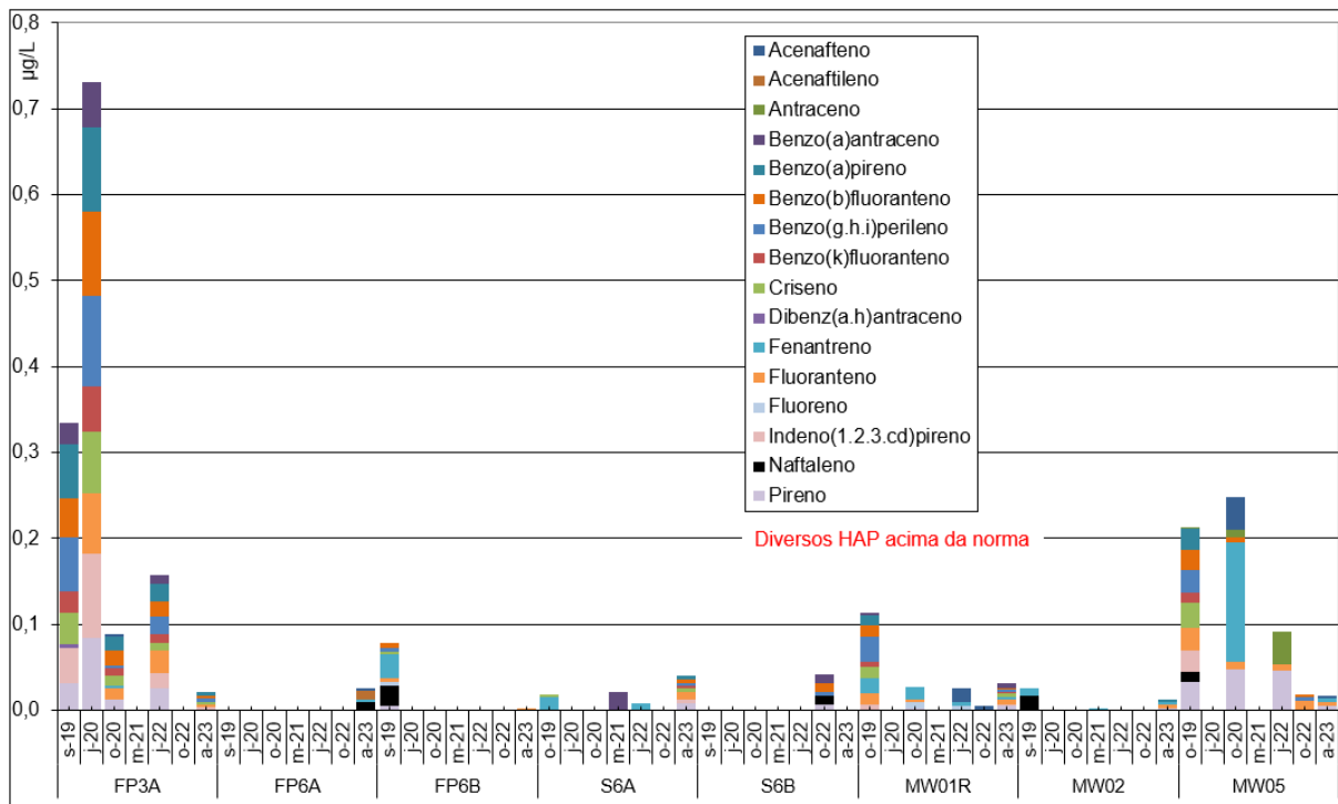
Figura 4.7 – Concentração em HAP na água de piezómetros localizados dentro e fora do Site 3001, entre 2019 e 2023
