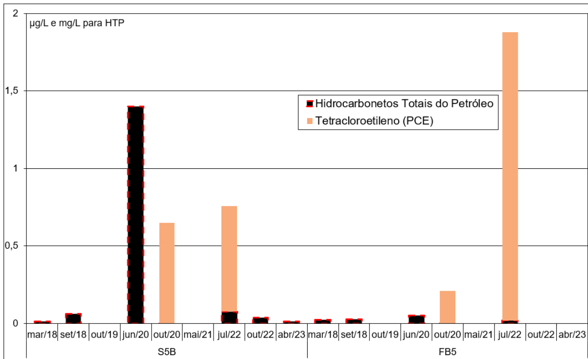
Figura 4.9 – Concentrações em HTP e PCE na água de piezômetros localizados fora do Site 5001, entre 2018 e 2023
