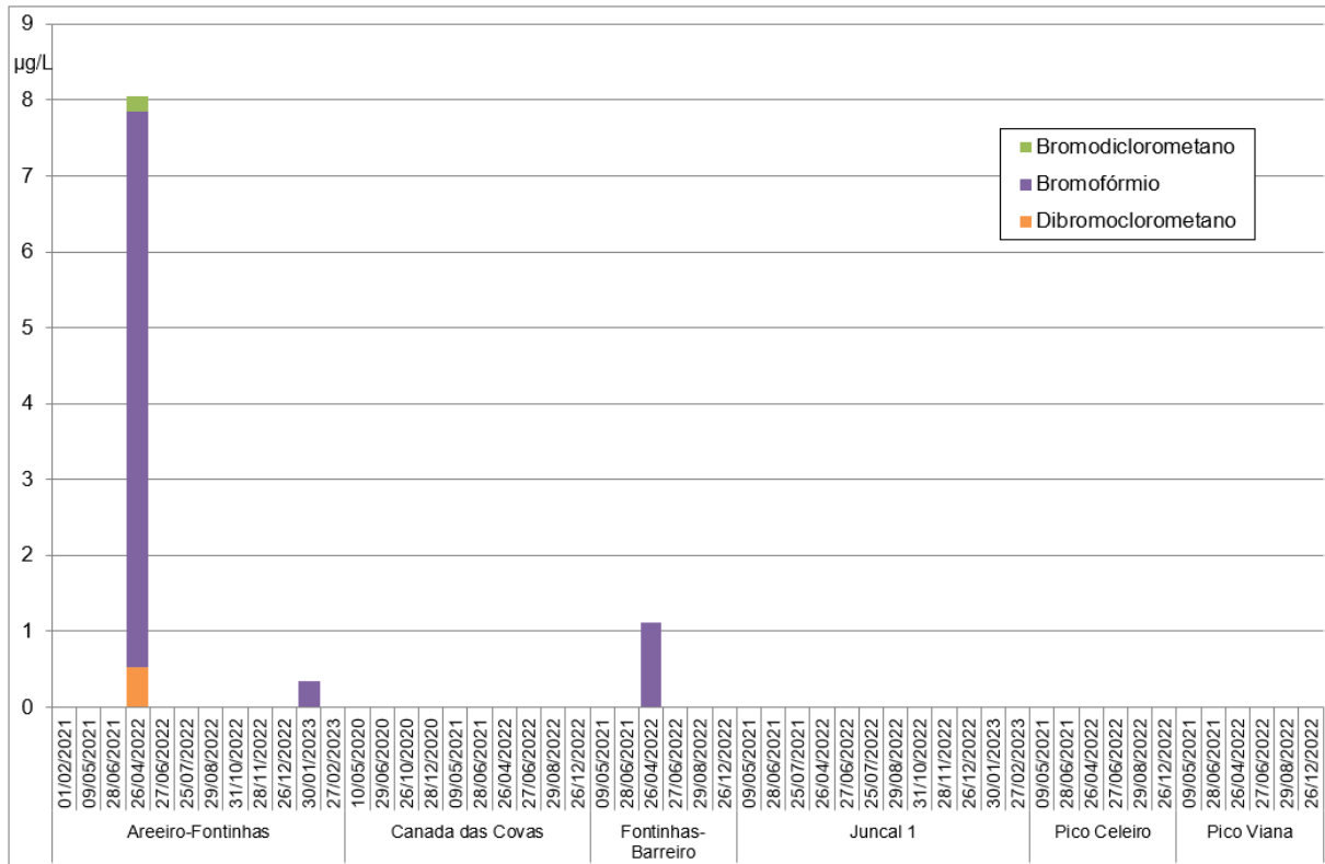
Figura 5.3 – Concentrações em COV nas águas subterrâneas dos furos de captação para eventual abastecimento público entre 2021 e 2023, para amostras pontuais
