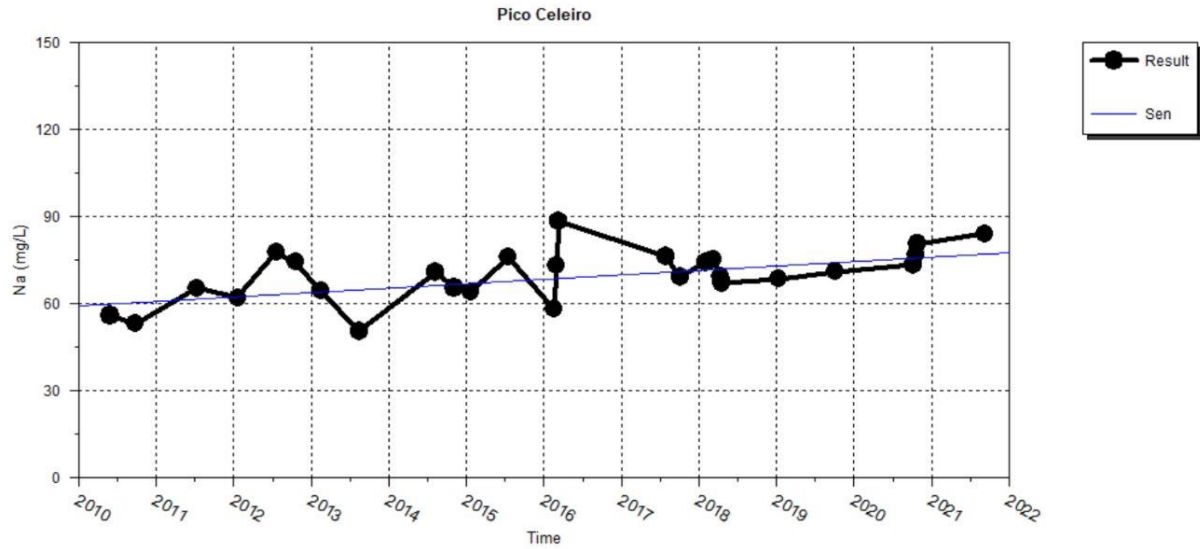
Figura 5.6 – Tendência crescente de sódio nas águas subterrâneas do furo do Pico Celeiro ("Sen" – traduz a magnitude da tendência)
