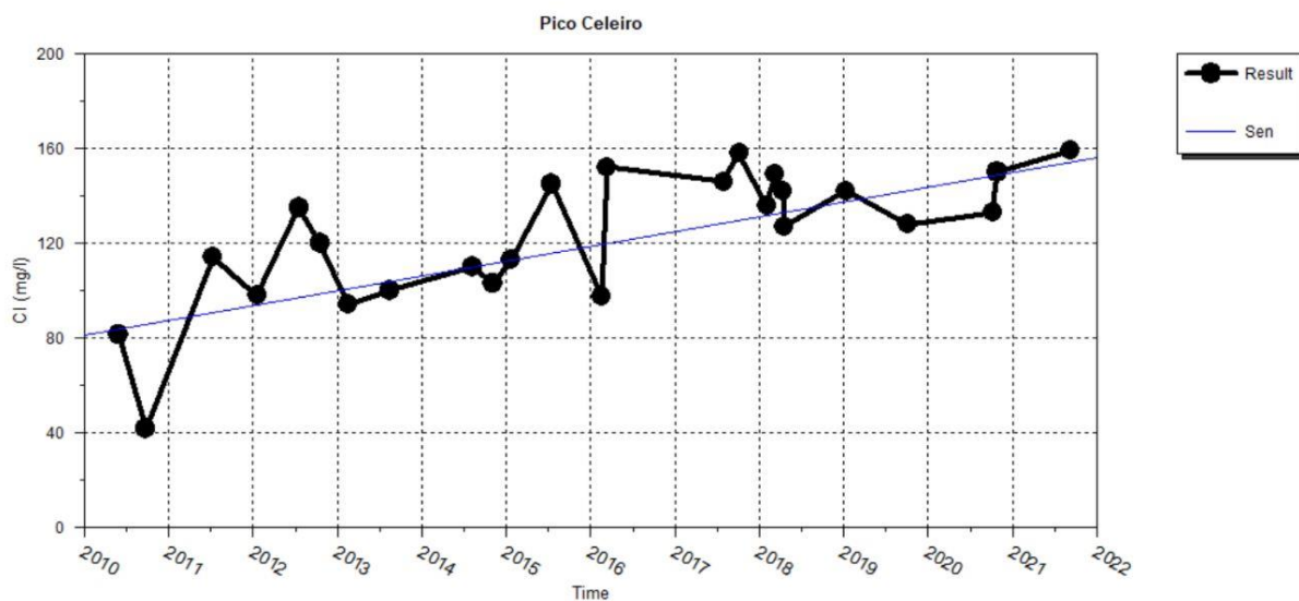
Figura 5.5 – Tendência crescente de cloretos nas águas subterrâneas do furo do Pico Celeiro ("Sen" – traduz a magnitude da tendência)
