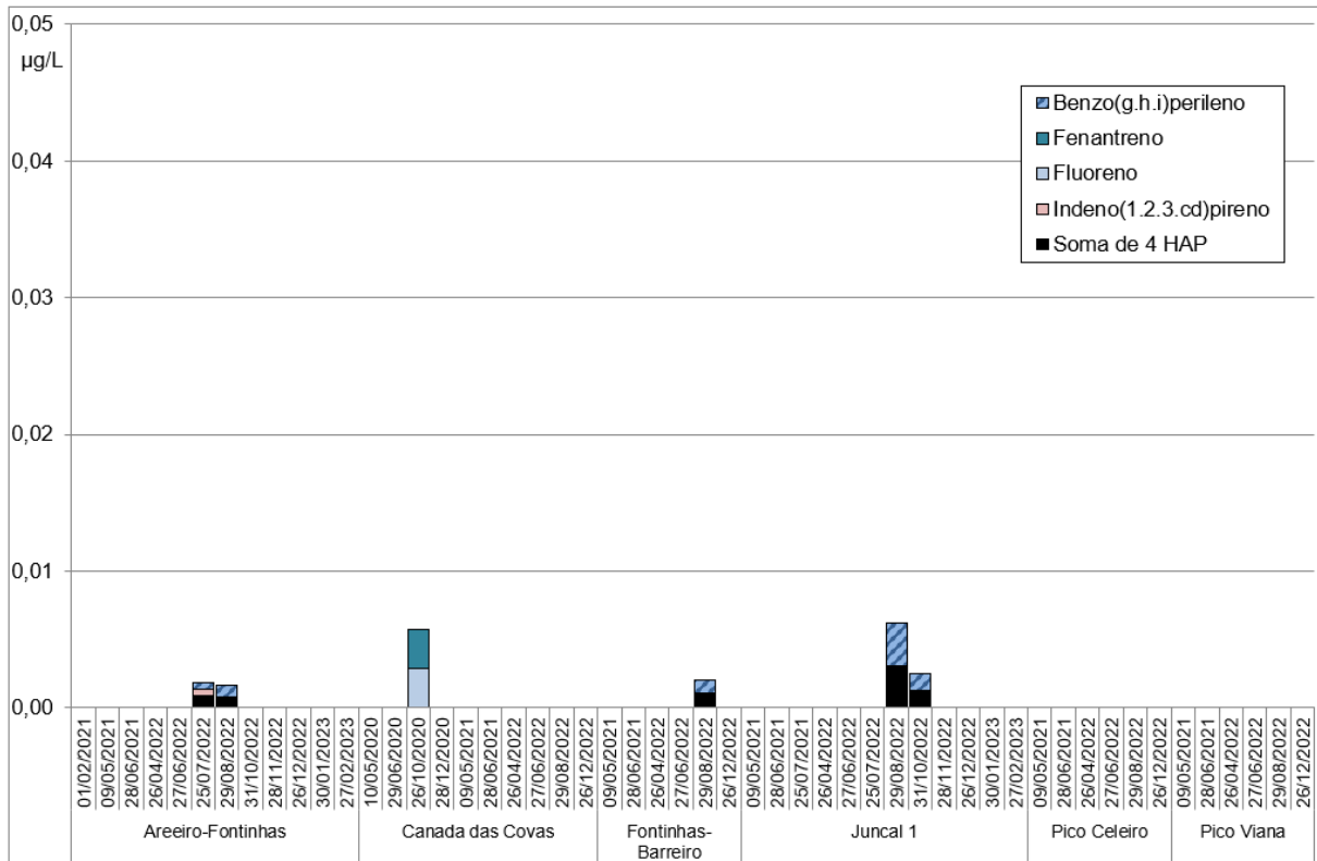
Figura 5.2 – Concentrações em HAP nas águas subterrâneas dos furos de captação para eventual abastecimento público entre 2021 e 2023, para amostras pontuais
