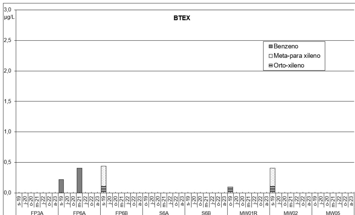
Figura 4.5 – Concentração em BTEX na água de piezómetros localizados dentro e fora do Site 3001, entre 2019 e 2023
