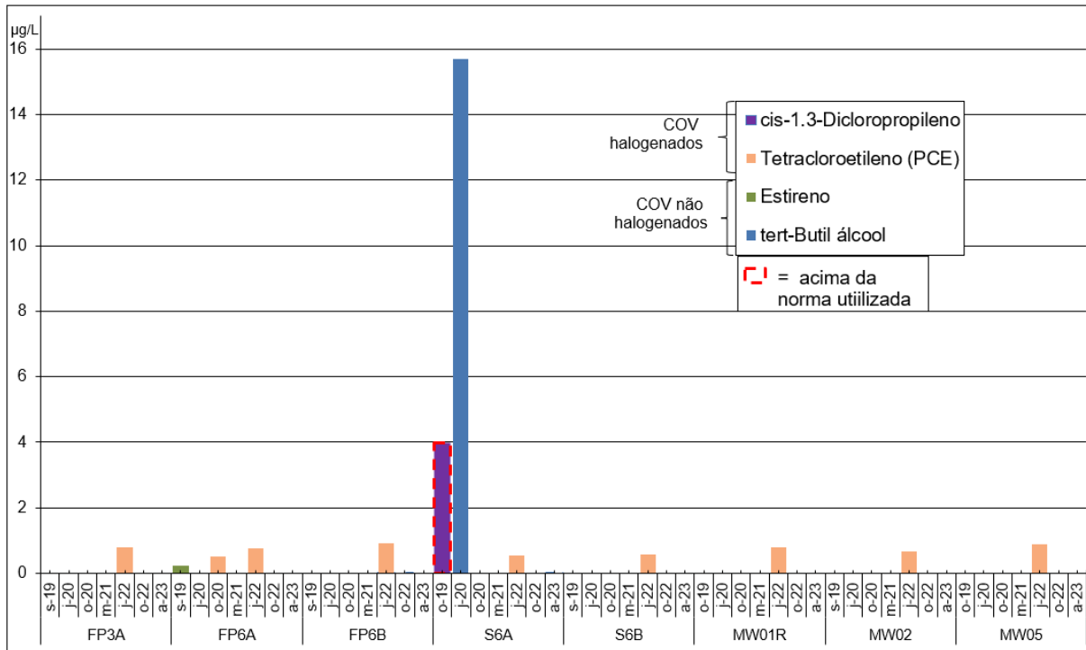
Figura 4.6 – Concentração em COV na água de piezómetros localizados dentro e fora do Site 3001, entre 2019 e 2023
