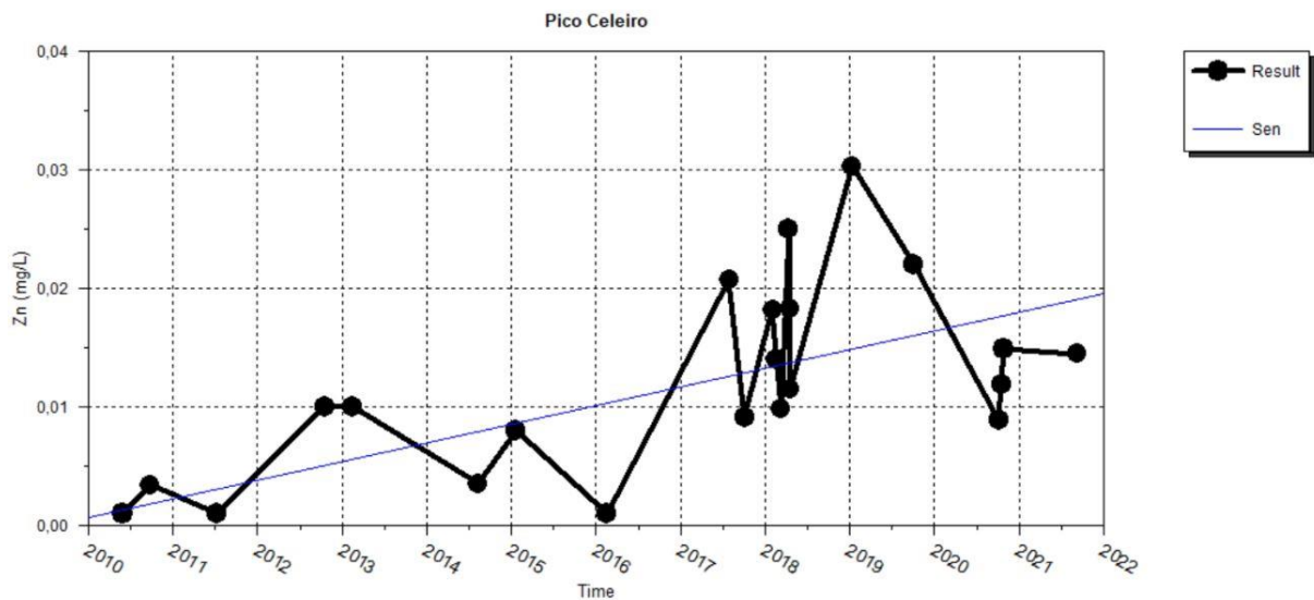
Figura 5.7 – Tendência crescente de zinco nas águas subterrâneas do furo do Pico Celeiro ("Sen" – traduz a magnitude da tendência)
