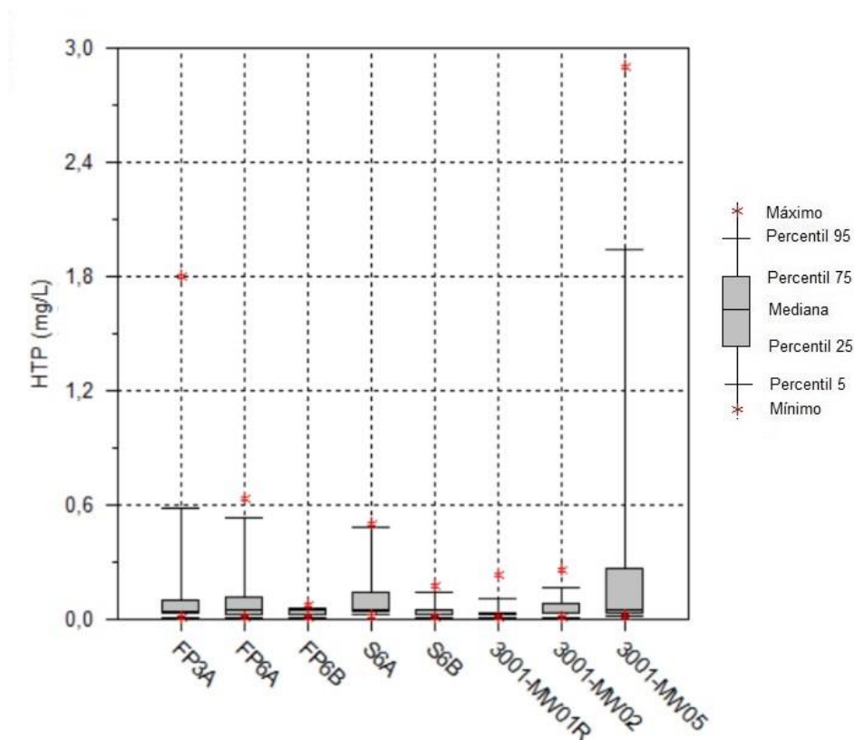
Figura 4.4 – Variação da concentração em HTP na água de piezómetros localizados dentro e fora do Site 3001, desde 2010
