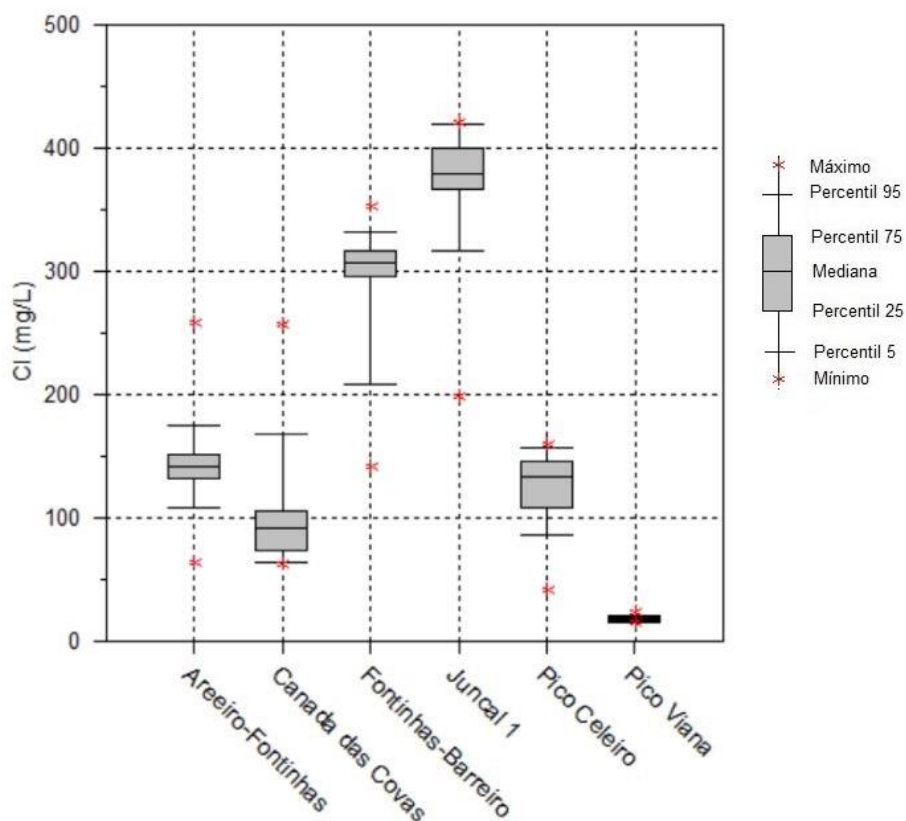
Figura 5.4 – Diagrama de box-plot das concentrações em cloreto nas águas subterrâneas dos furos de captação para eventual abastecimento público
