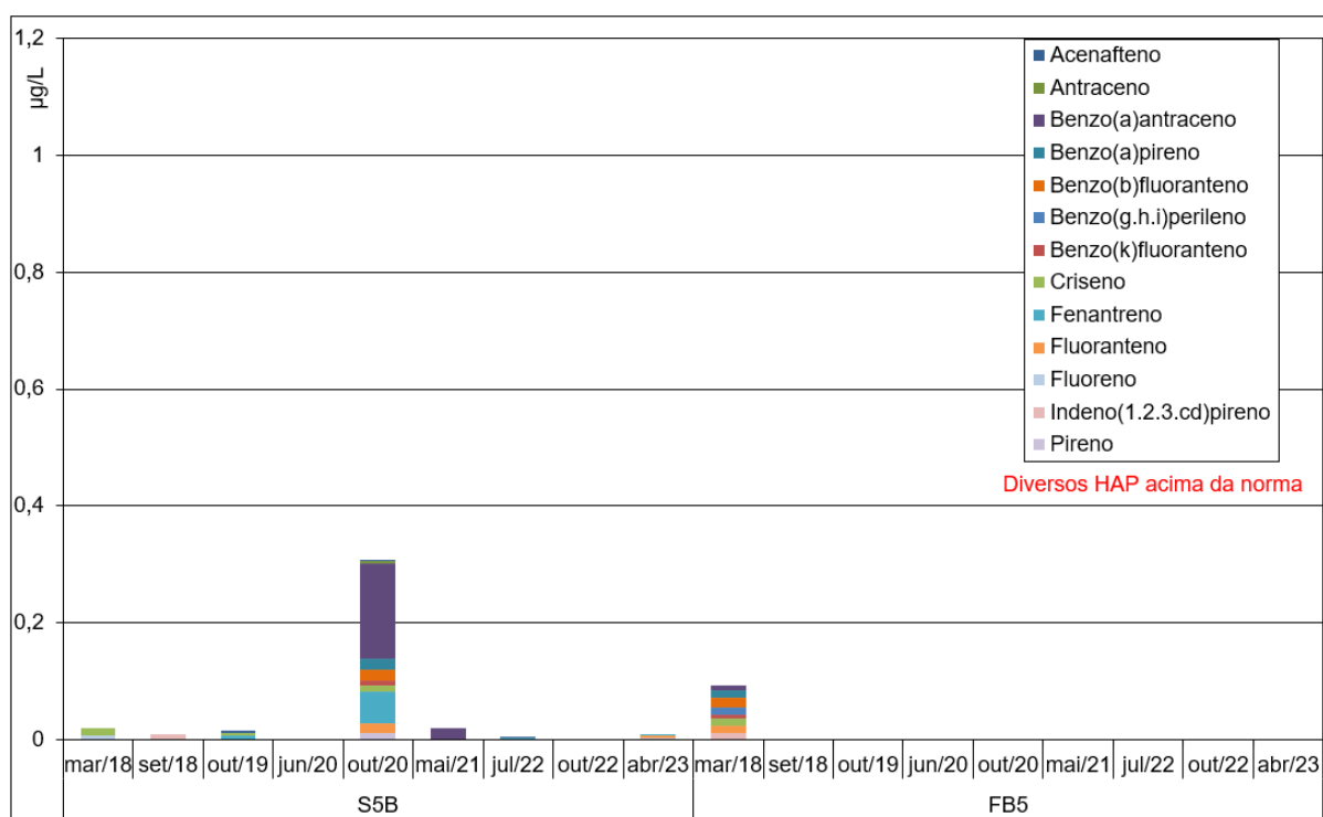
Figura 4.10 – Concentrações em HAP na água de piezómetros localizados fora do Site 5001, entre 2018 e 2023
