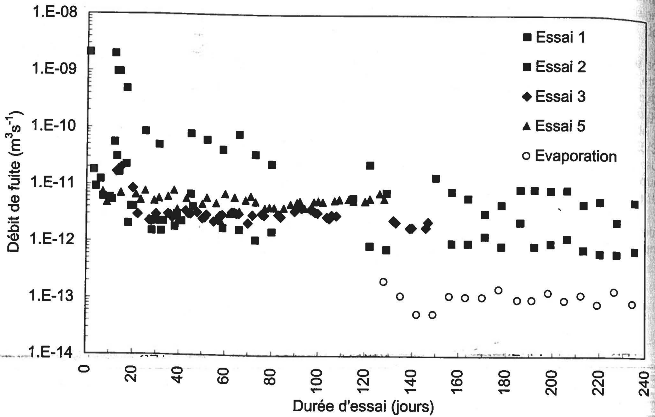
Figure 3. Evolution temporelle des débits de fuite mesurés pour les essais 1, 2, 3 et 5 comparés à l'évaporation
