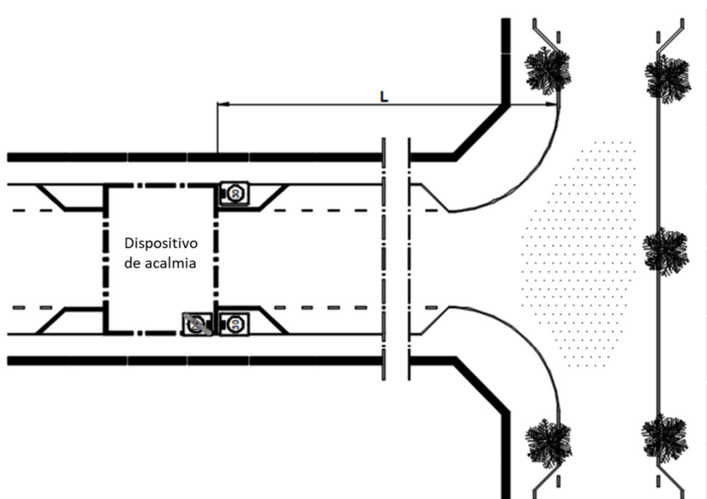
Figura 3.9 – Solução para limites de Zonas 30 em secção corrente (CROW, 1998)
