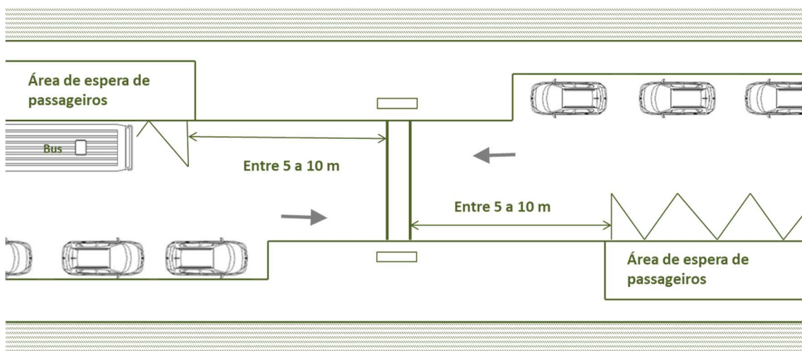
Figura 5.11 – Configuração de paragem com estacionamento alternado (SMTC Tisséo, 2016)
