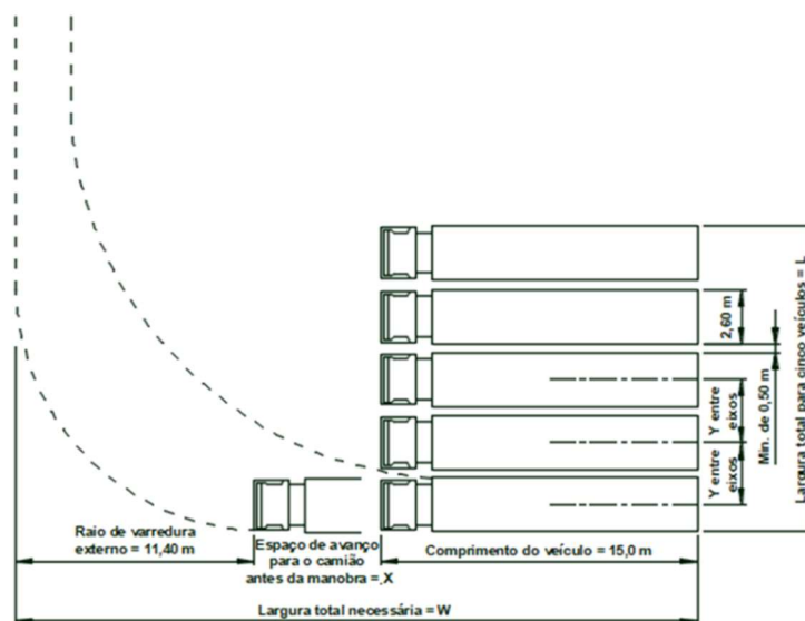
Figura 6.10 – Estacionamento perpendicular de veículos pesados de mercadorias de grande dimensão considerando a área de varredura (adaptado de Littlefield, D., 2011)
