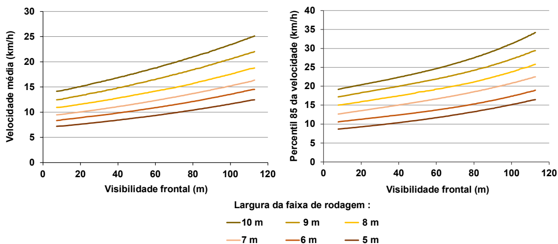
Figura 2.6 – Velocidades de circulação, em função da largura da rua e da distância de visibilidade para a frente (Adaptado de York et al. , 2007).
