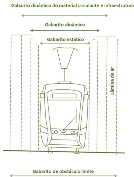
Figura 5.2 – Largura do elétrico (CEREMA, 2016)
