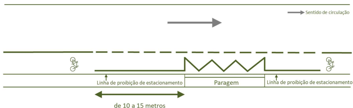
Figura 5.13 – Localização da paragem na proximidade de pistas para bicicletas (CEREMA, 2018)
