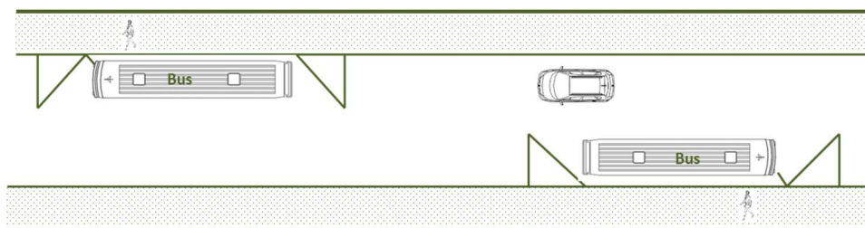
Figura 5.6 – Configuração de paragens em linha em arruamento sem estacionamento de veículos na área adjacente – Tipo A-2 (adaptado de CEREMA, 2016)
