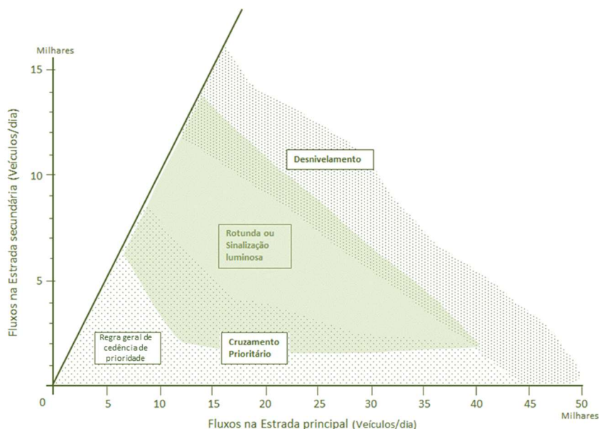
Figura 2.7 – Tipologia de cruzamentos admissíveis e sua capacidade potencial (adaptado de Seco et al. , 2008c).
