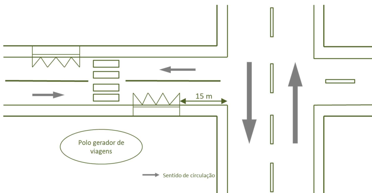
Figura 5.10 – Configuração de paragem de autocarro junto a intersecção (CEREMA, 2018)
