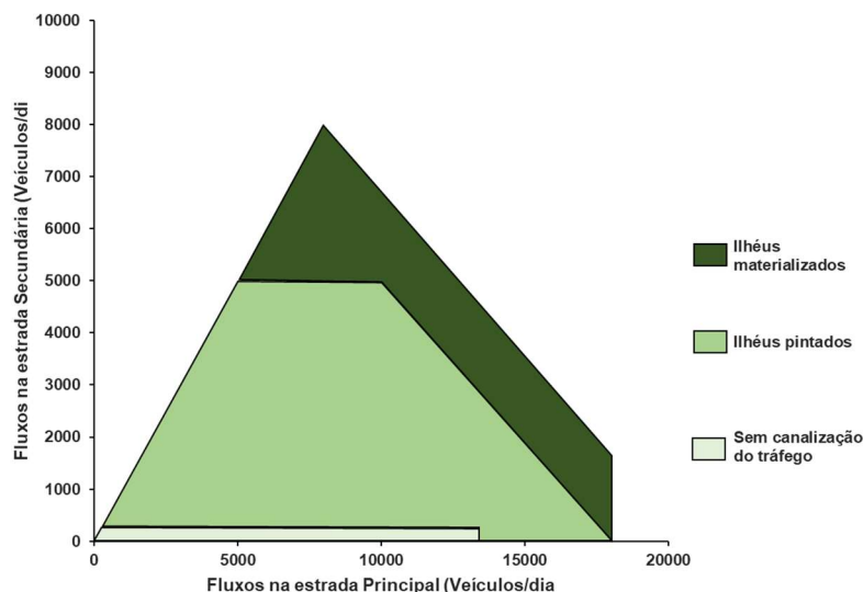
Figura 3.5 – Domínio de aplicação privilegiado das intersecções prioritárias (Department for Transport, 1995, referido em Silva, et al. , 2011b)
