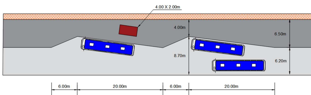
Figura 5.16 – Configuração geométrica de uma estação terminal de autocarros (SMTC Tisséo, 2016)
