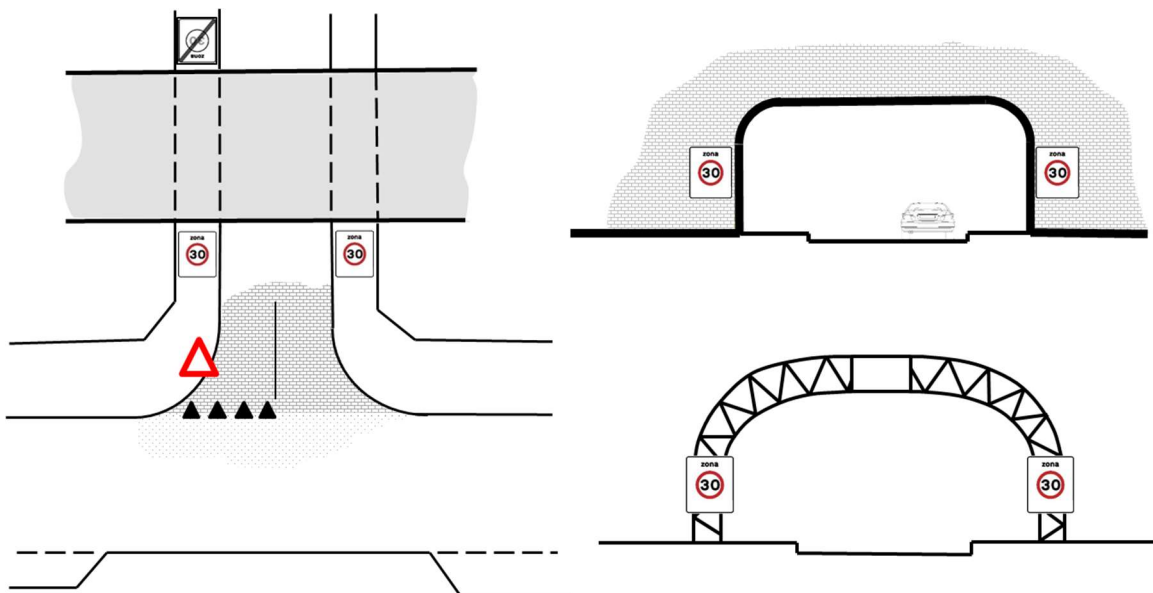
Figura 3.8 – Solução para limites de Zonas 30 com arcos ou edificações (CROW, 1998)
