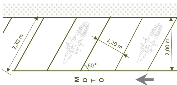
Figura 6.7 – Estacionamento oblíquo de motos (adaptado de CEREMA, 2016)
