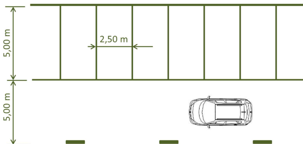
Figura 6.4 – Estacionamento perpendicular (adaptado de CEREMA, 2016)
