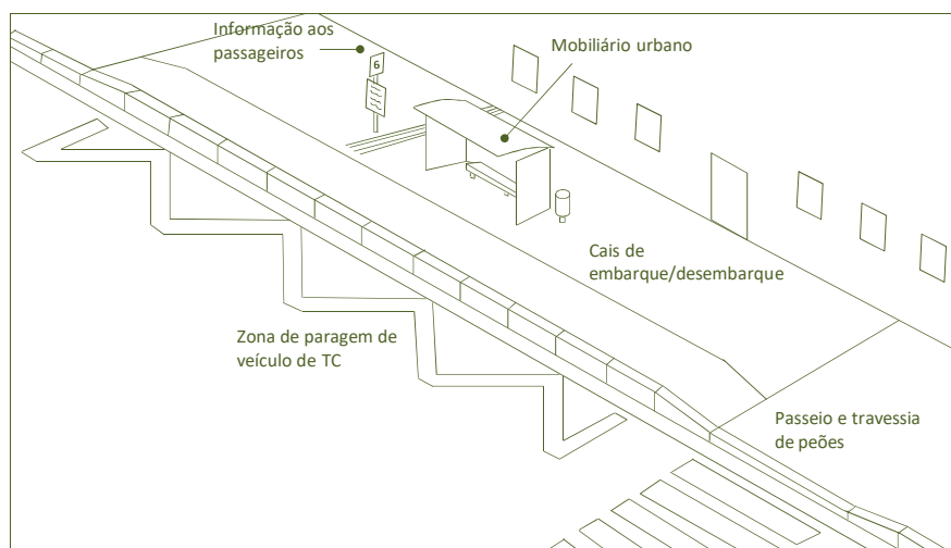
Figura 5.15 – Paragem de autocarro acessível com abrigo (adaptado de CEREMA, 2018)
