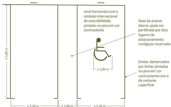
Figura 6.6 – Dimensões dos lugares acessíveis contíguos (SNRIPD, 2006)
