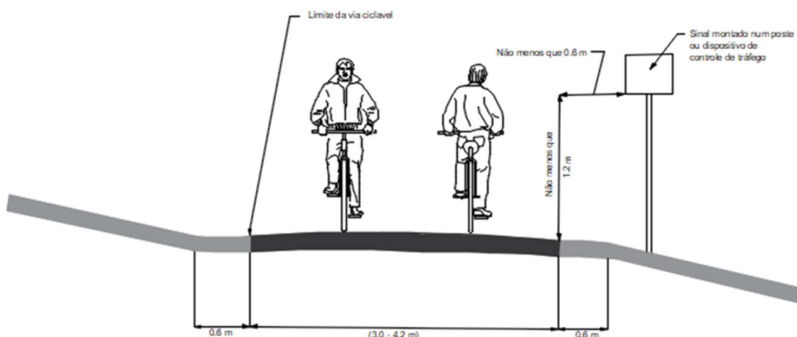
Figura 2.2 – Perfil transversal tipo de pistas cicláveis bidirecionais (adaptado de AASHTO, 2012).
