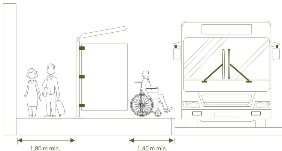
Figura 5.3 – Configuração de paragem de autocarro acessível.
