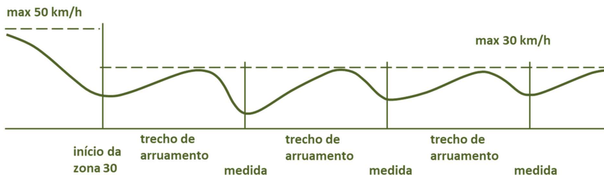
Figura 4.2 – Perfil de velocidades desejado numa Zona 30
