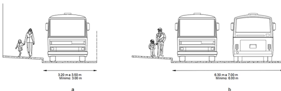
Figura 5.1 – Largura de vias bidirecionais (a) e unidirecionais (b) reservadas ao TC de passageiros (adaptado de CEREMA, 2016)
