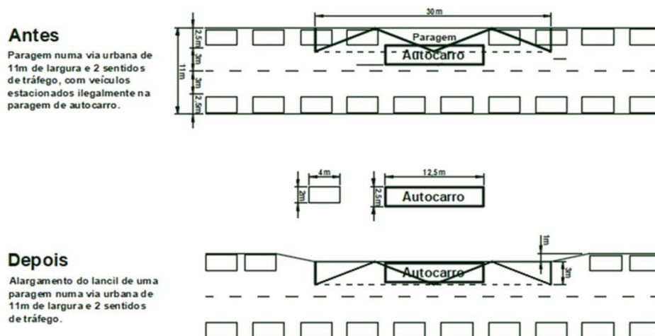
Figura 5.14 – Medida para prevenir o estacionamento ilegal em paragem avançada de autocarro (Seco, A. et al., 2008)
