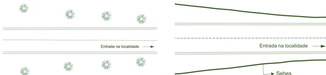
Figura 3.4 – Disposição recomendada dos elementos verticais na aproximação do portão de entradas da zona urbana (adaptado de Silva, et al. , 2011b)
