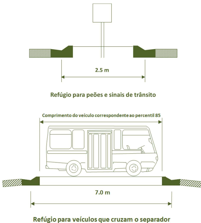
Figura 2.4 – Exemplo de separador central com lancil (adaptado de AASHTO, 2012)
