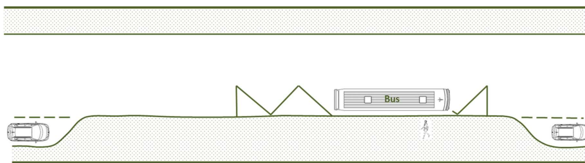
Figura 5.7 – Configuração de uma paragem sem estacionamento de veículos na área adjacente – Tipo B (adaptado de CEREMA, 2016)
