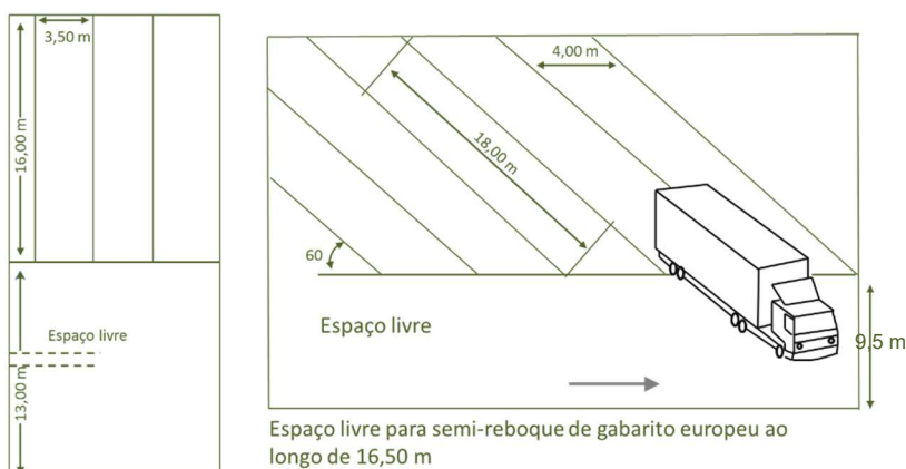
Figura 6.9 – Estacionamento de veículos pesados de mercadorias (INRS, 2010)
