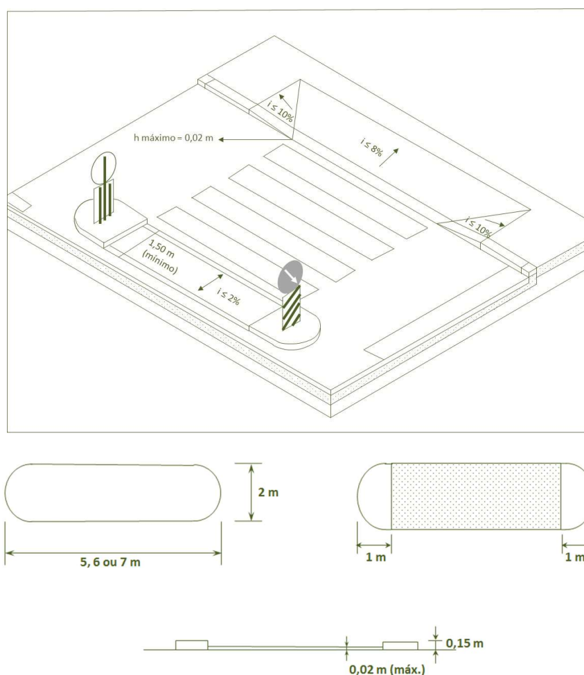
Figura 2.5 – Dimensões de refúgio para peões (adaptado de SNRIPD, 2006 e Seco, et al. , 2008b).
