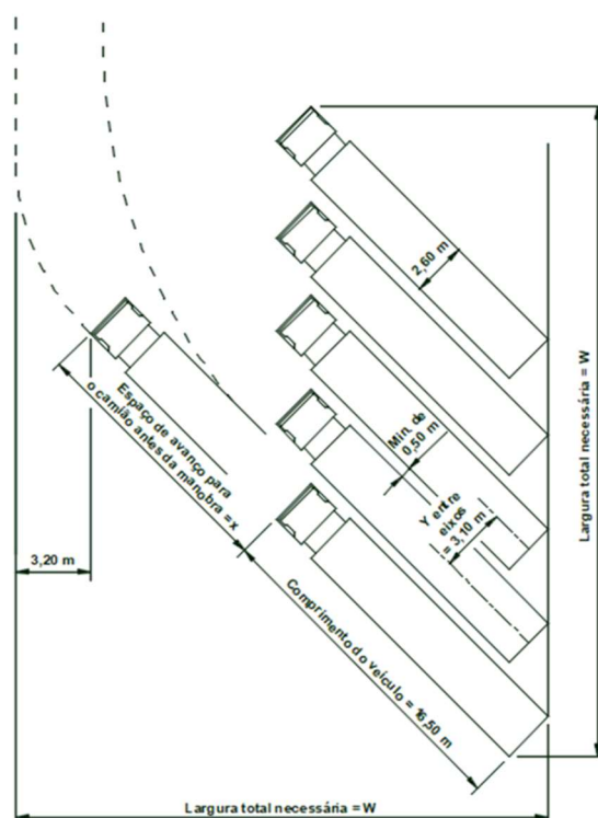
Figura 6.11 – Estacionamento oblíquo de veículos pesados de mercadorias de grande dimensão (adaptado de Littlefield, D., 2011)
