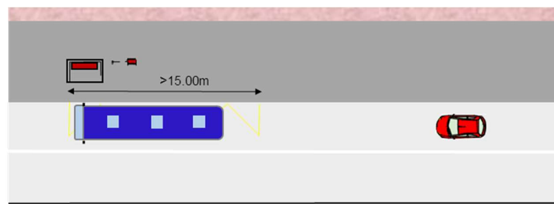
Figura 5.5 – Configuração de uma paragem em linha sem estacionamento adjacente - Tipo A-1 (SMTCC Tisséo, 2016)
