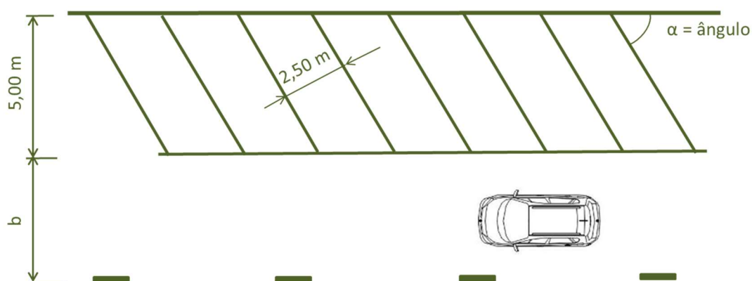
Figura 6.5 – Estacionamento oblíquo (adaptado de CEREMA; 2016)
