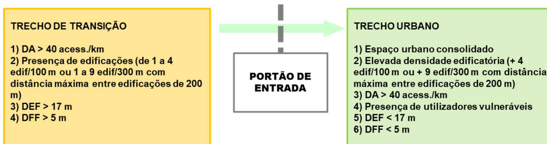
Figura 3.2 – Localização de portão de entrada em trecho de atravessamento de espaço urbano (Silva et al. , 2011a)
