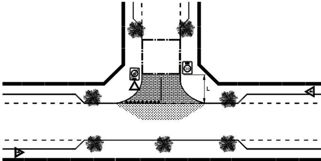
Figura 3.7 – Solução simples para limites de Zonas 30 (CROW, 1998)
