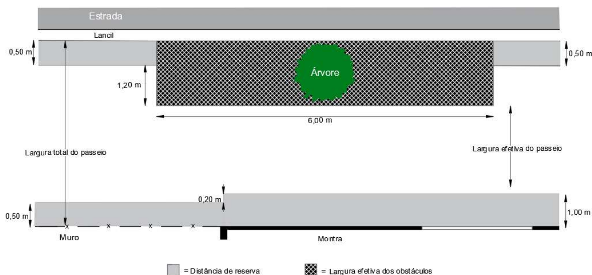
Figura 2.3 – Exemplo de distâncias de reserva e larguras efetivas de obstáculos (adaptado de TRB, 2010)
