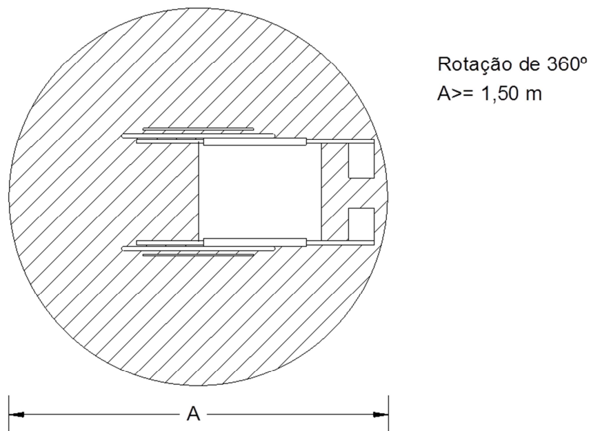
Figura 3.11 – Espaço de manobra de uma cadeira de rodas (SNRIPD, 20016)
