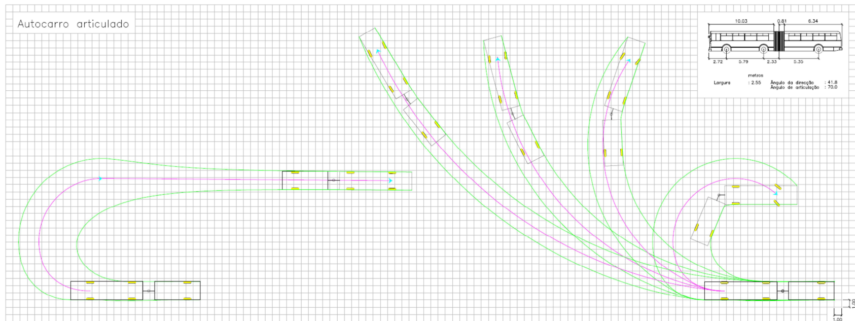
Figura A1.7 – Áreas de varredura de um autocarro articulado (Macedo et al. , 2011).
