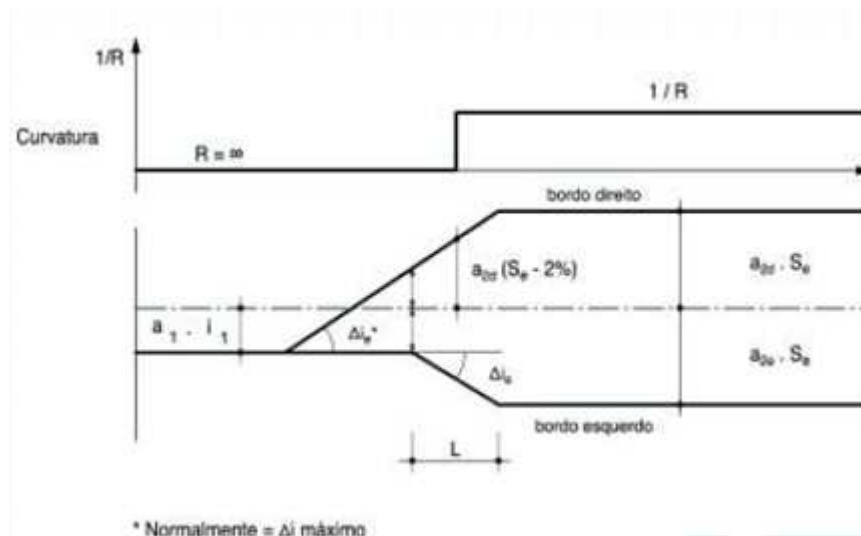
Figura 5.7 – Transição da sobrelevação sem curva de transição (trabalho de revisão da Norma de Traçado, referido em Macedo e Cardoso, 2010)
