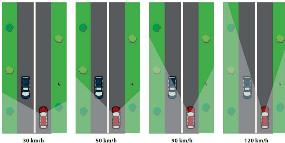
Figura 3.4 – Características do campo visual para várias velocidades (Babkov, 1987 4 , citado em ACEM, 2006)
