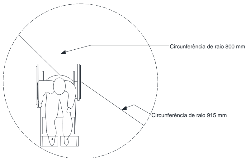
Figura 3.10 – Espaço de manobra de uma cadeira de rodas (Austroads, 2017c)
