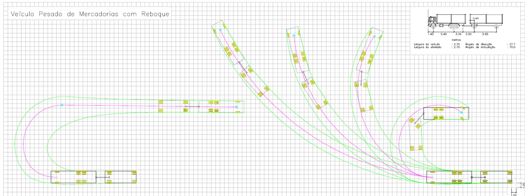
Figura A1.4 – Áreas de varredura de um veículo pesado de mercadorias com reboque (Macedo et al., 2011).
