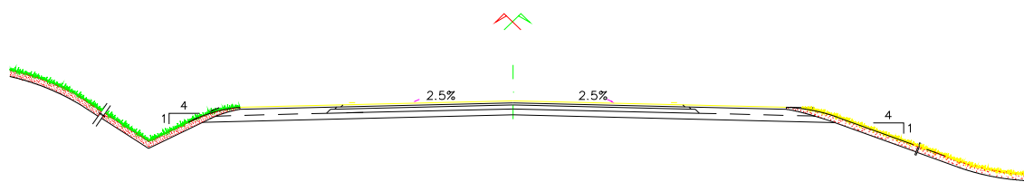
a) Perfil transversal em reta
