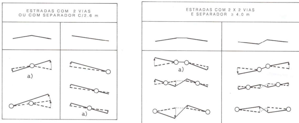
Figura 5.8 – Exemplos de eixos de rotação (JAE, 1994).
