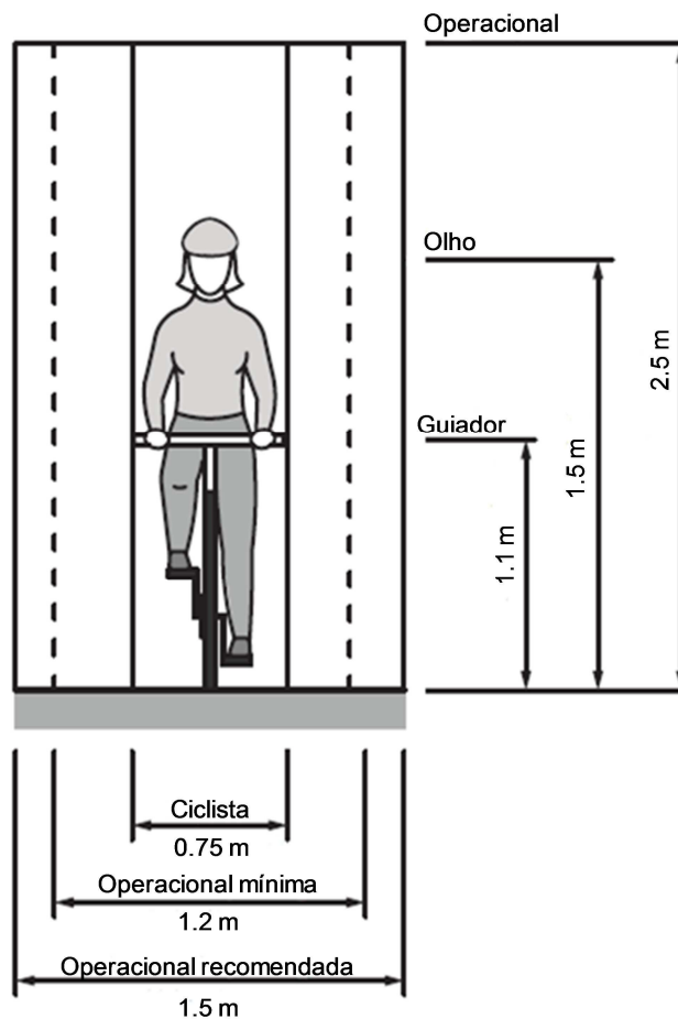
Figura 3.16 – Espaço de manobra de um ciclista (AASHTO, 2012).
