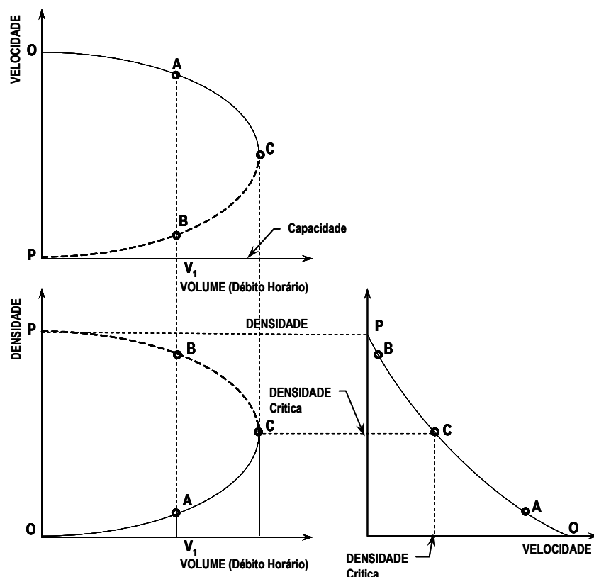
Figura 4.4 – Relações entre Velocidade, Volume e Densidade de Tráfego (Macedo, Cardoso e Roque, 2011).
