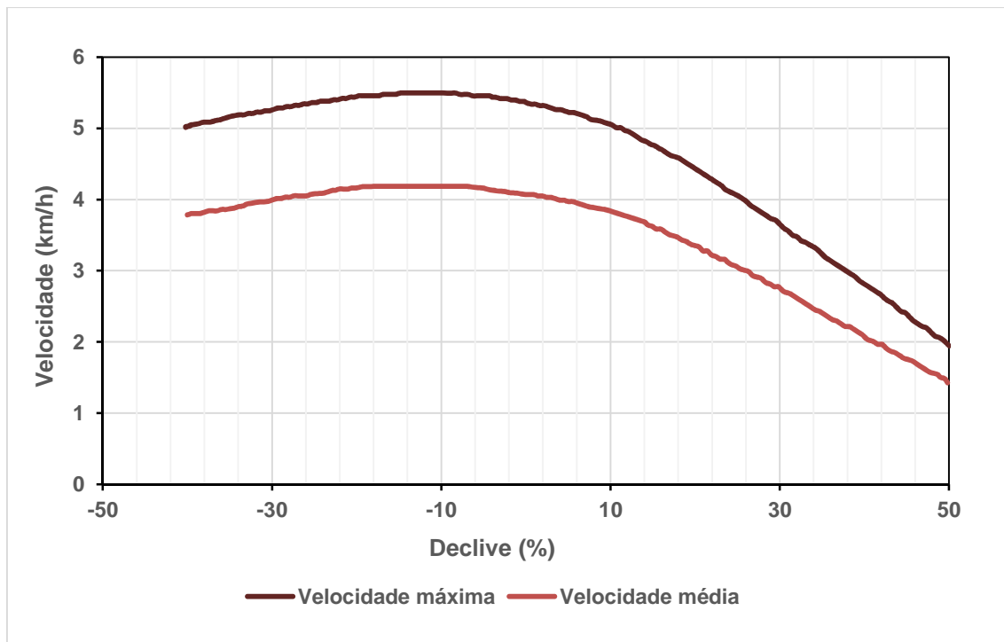
Figura 3.13 – Velocidade de circulação do peão em função do declive (EPFL-LITEP 11 , 1995, referido em IMTT, I.P., 2011a)
