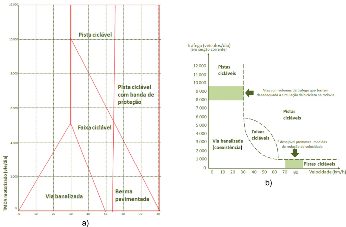
Figura 5.13 – Seleção do tipo de percurso ciclável (adaptado de Veidirectoratet, 2000 e CERTU, 1998)
