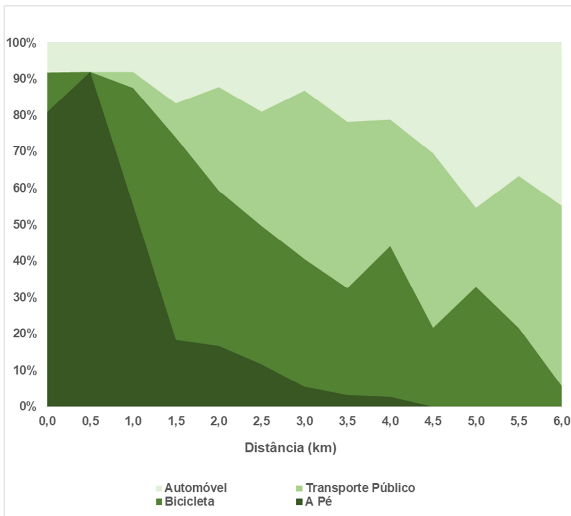
Figura 3.14 – Repartição modal típica em função do comprimento da viagem (Pita, 2002 12 , referido em Seco, Macedo e Pires da Costa, 2008)
