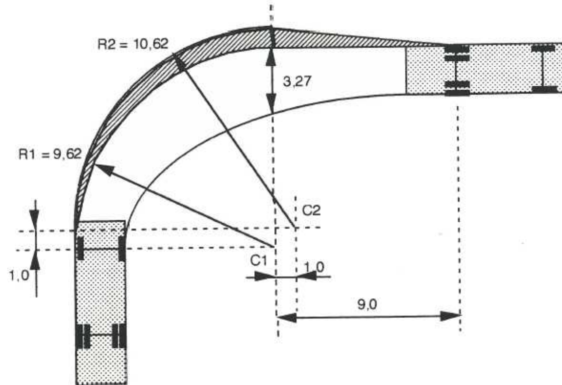
Figura A1.8 – Áreas de varredura de um veículo tipo de recolha de resíduos sólidos urbanos (Campos, 1993).
