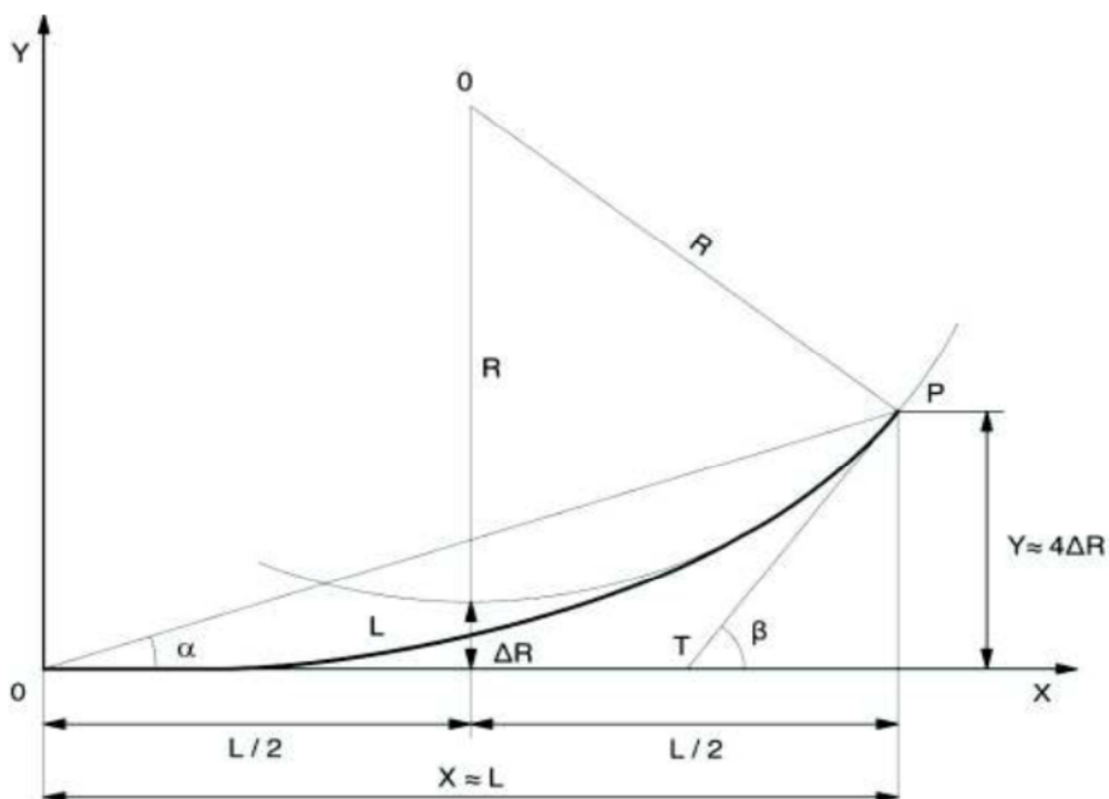
Figura 5.3 – Representação esquemática de uma clotoide no seu referencial próprio (trabalho de revisão da Norma de Traçado, referido em Macedo e Cardoso, 2010)
