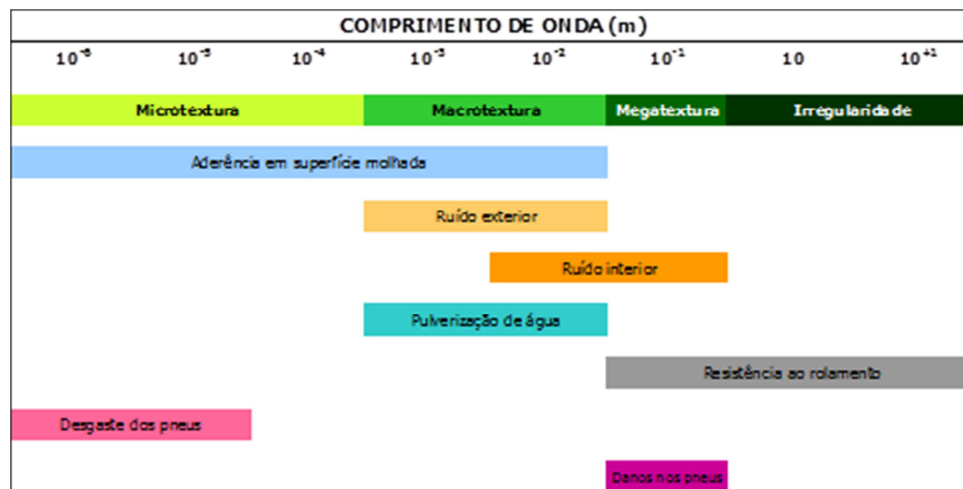
Figura 3.24 – Classificação das características superficiais segundo a AIPCR (PIARC, 1987).
