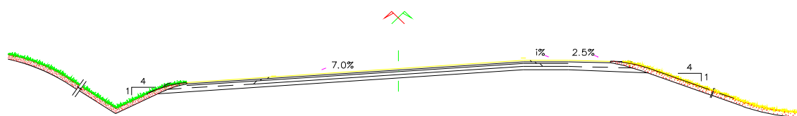
b) Perfil transversal em curva com sobrelevação
