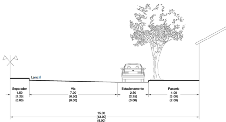
Figura 5.12 – Elementos do perfil transversal de uma rodovia urbana sem condicionamento de acessos (adaptado de Seco et al. , 2008).
