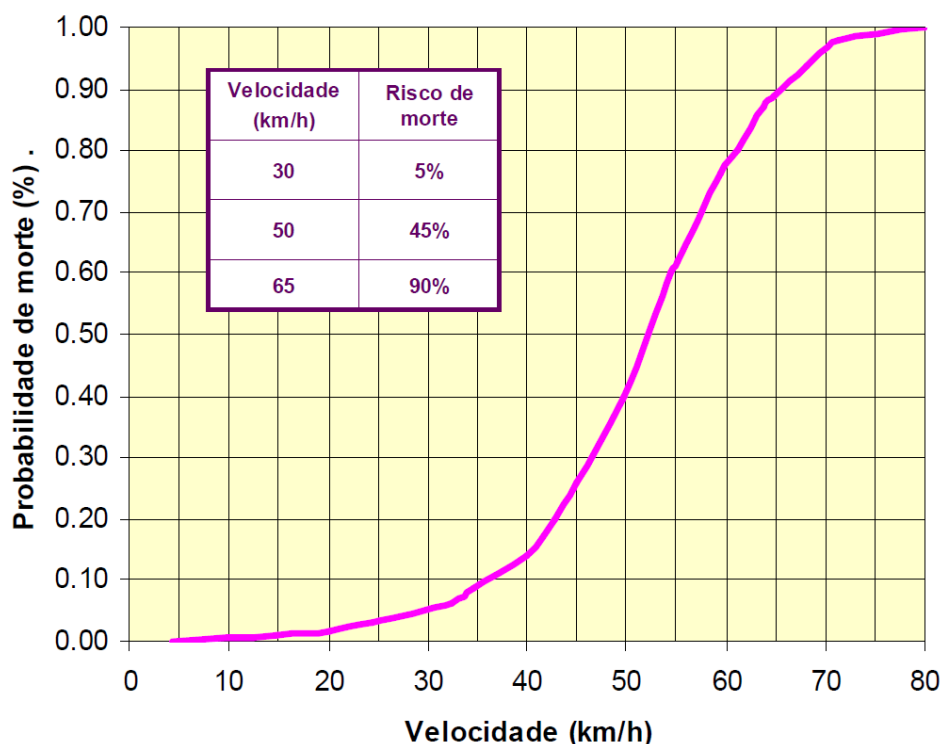
Figura 3.15 – Risco de morte de peão, por atropelamento, em função da velocidade do veículo (Cardoso, 2001)
