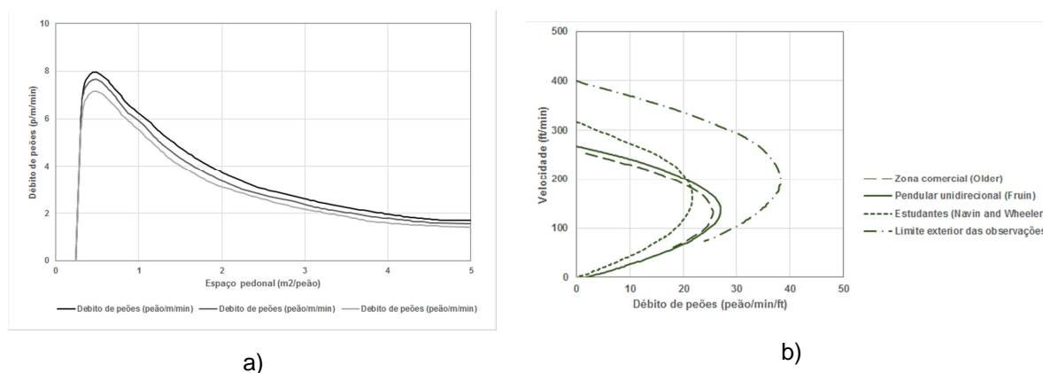
Figura 4.8 – Relação entre volume, densidade e velocidade de peões (TRB, 2018)
