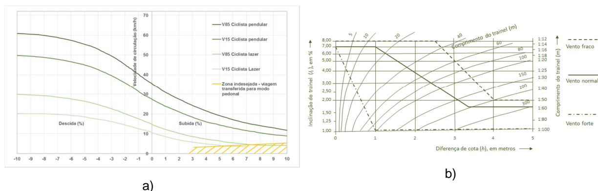
Figura 5.9 – Impactes dos trainéis na circulação de bicicletas (adaptado de CROW, 1998).
