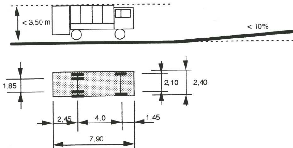
Figura 3.20 – Dimensões do veículo tipo de recolha de resíduos sólidos urbanos (Campos, 1993).
