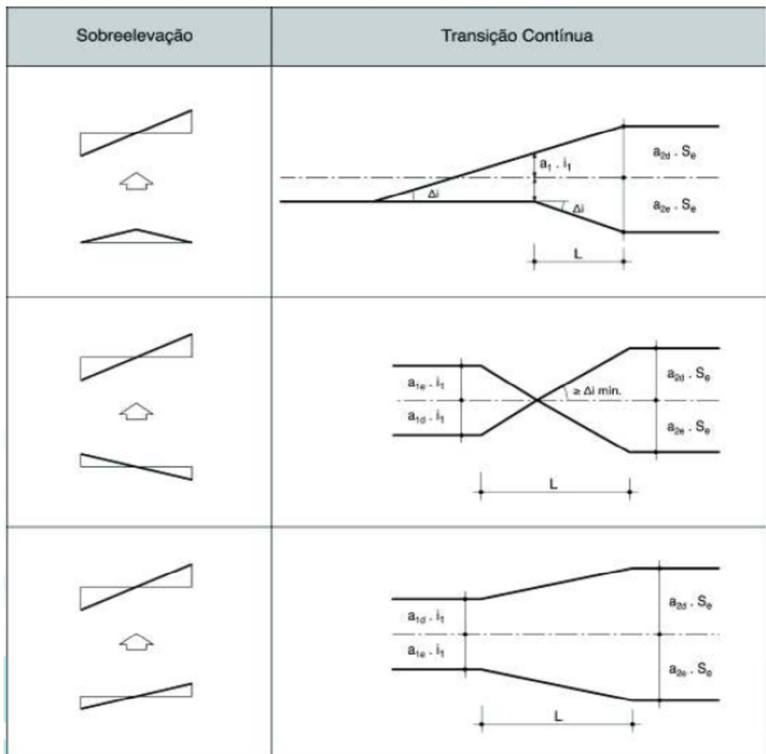
Figura 5.6 – Transição da sobrelevação com curva de transição (trabalho de revisão da Norma de Traçado, referido em Macedo e Cardoso, 2010)
