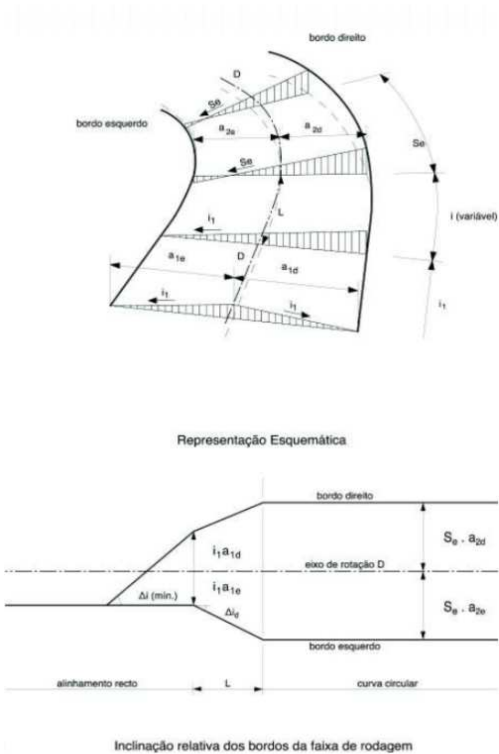
Figura 5.4 – Transição da sobrelevação (rotação em torno do eixo) (JAE, 1994)
