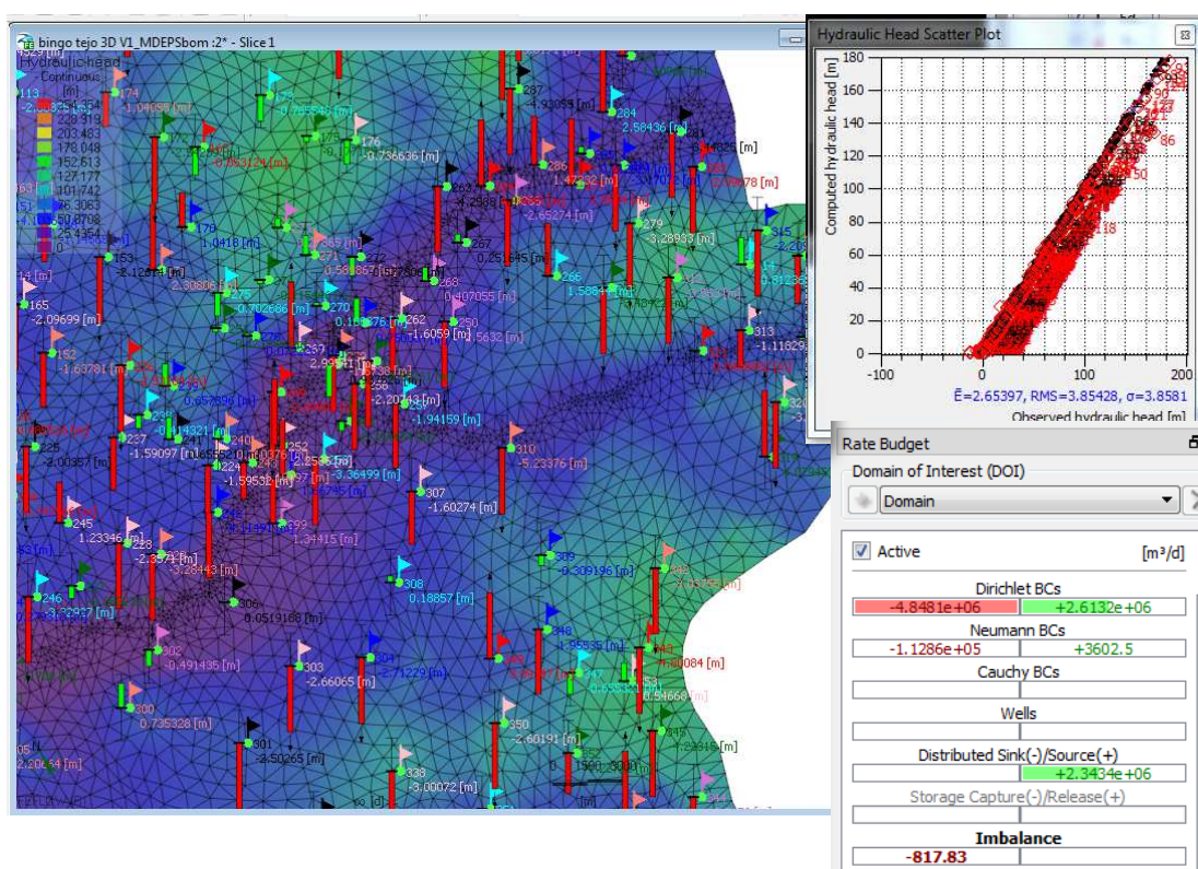
Figura 9. Calibração para condições naturais, regime permanente, com erro de balanço e gráfico de ajustamento dos valores observados/simulados
