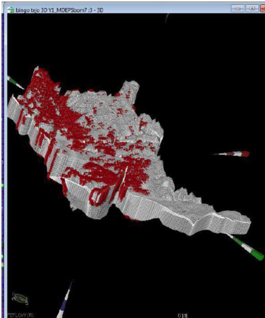
Figura 8. Furos de extracção
