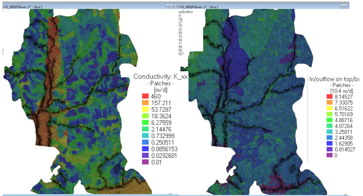
Figura 6. Distribuição das condutividades hidráulicas após calibração
