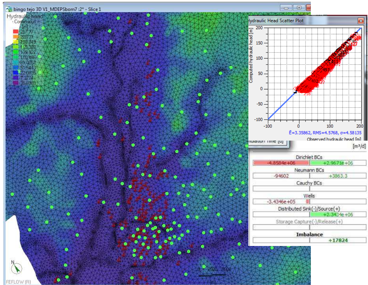
Figura 10. Calibração para condições de bombagem, regime permanente, com a distribuição dos furos de captação, erro de balanço e gráfico de ajustamento dos valores observados/simulados
