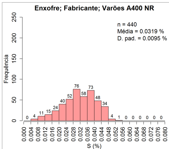
Figura 25: Valores do teor de enxofre do aço A400 NR obtidos pelos Fabricantes
