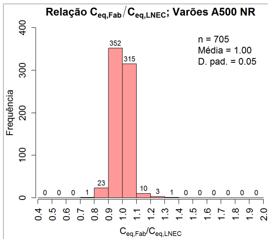
Figura 18: Relação entre carbono equivalente do A500 NR obtidos pelos Fabricantes e pelo LNEC
