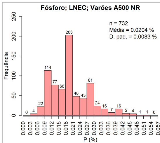
Figura 36: Valores do teor de fósforo do aço A500 NR obtidos pelo LNEC
