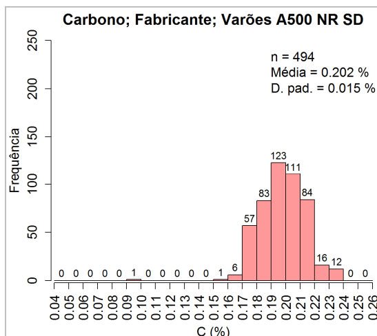
Figura 8: Valores do teor de carbono do aço A500 NR SD obtidos pelos Fabricantes
