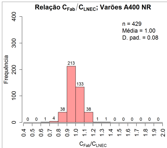
Figura 5: Relação entre teores de carbono do aço A400 NR obtidos pelos Fabricantes e pelo LNEC
