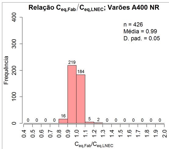
Figura 17: Relação entre carbono equivalente do A400 NR obtidos pelos Fabricantes e pelo LNEC
