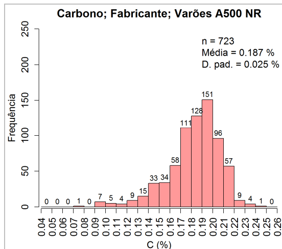
Figura 2: Valores do teor de carbono do aço A500 NR obtidos pelos Fabricantes
