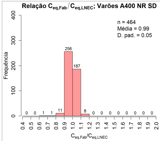
Figura 23: Relação entre carbono equivalente do A400 NR SD obtidos pelos Fabricantes e pelo LNEC
