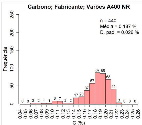
Figura 1: Valores do teor de carbono do aço A400 NR obtidos pelos Fabricantes
