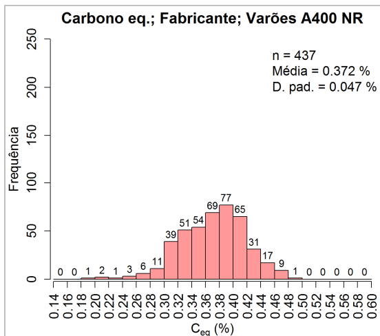
Figura 13: Valores do teor de carbono equivalente do aço A400 NR obtidos pelos Fabricantes
