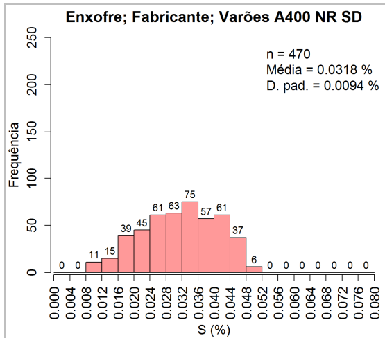
Figura 29: Valores do teor de enxofre do aço A400 NR SD obtidos pelos Fabricantes
