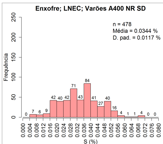
Figura 31: Valores do teor de enxofre do aço A400 NR SD obtidos pelo LNEC
