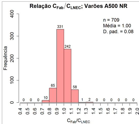
Figura 6: Relação entre teores de carbono do aço A500 NR obtidos pelos Fabricantes e pelo LNEC
