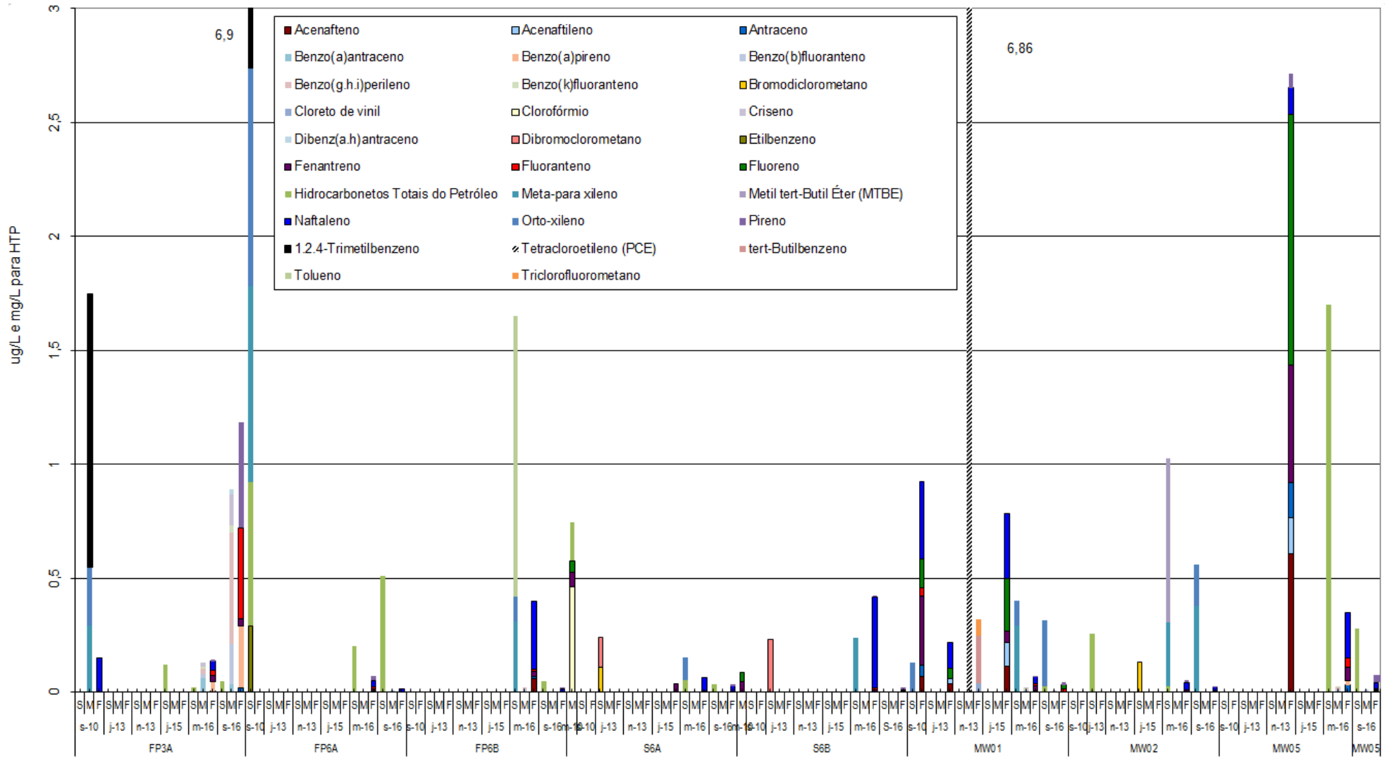
Figura 4.2 – Concentração em PAH, TPH e BTEX em oito piezómetros localizados nas formações hidrogeológicas superficial e intermédia, dentro e fora do Site 3001, entre 2010 e 2016
