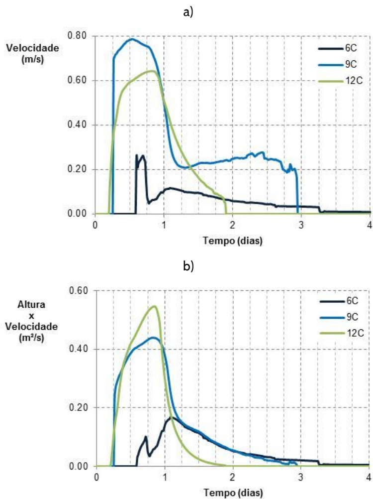
Figura 11 - Velocidade (a) e produto da altura pela velocidade (b) nos pontos 12C, 9C e 6C para o cenário III.
