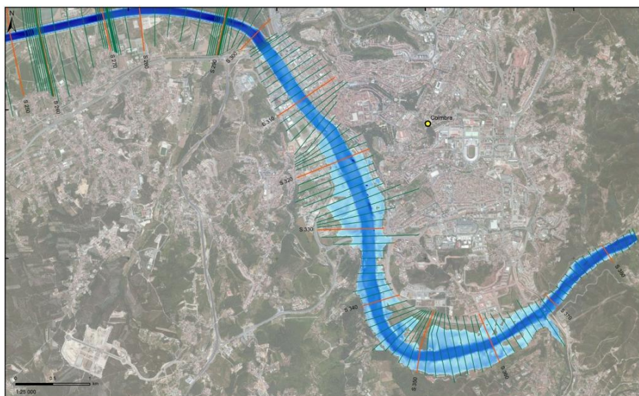
Figura 8 - Zonas inundáveis junto a Coimbra para o cenário II.
