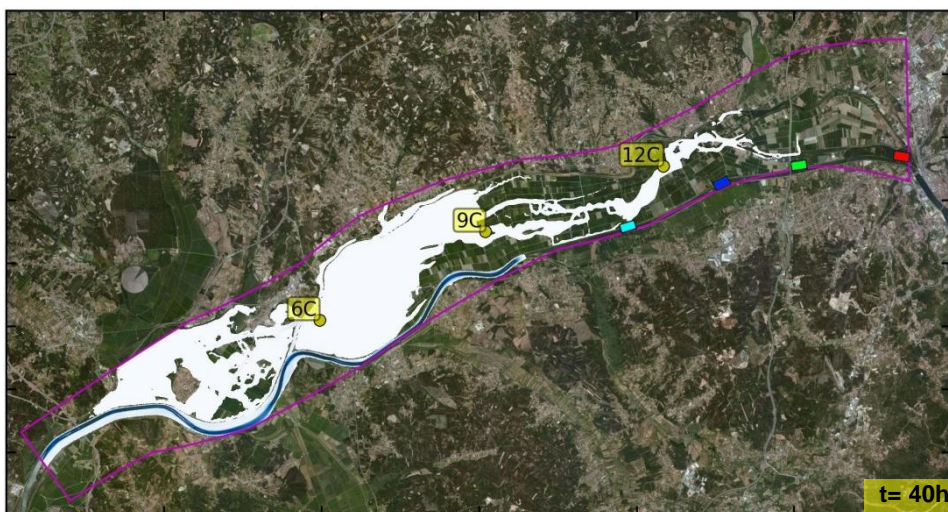
Figura 9 - Inundações na margem direita do rio Mondego em vários instantes de tempo originadas pelo sistema de inundação controlada (cenário III).
