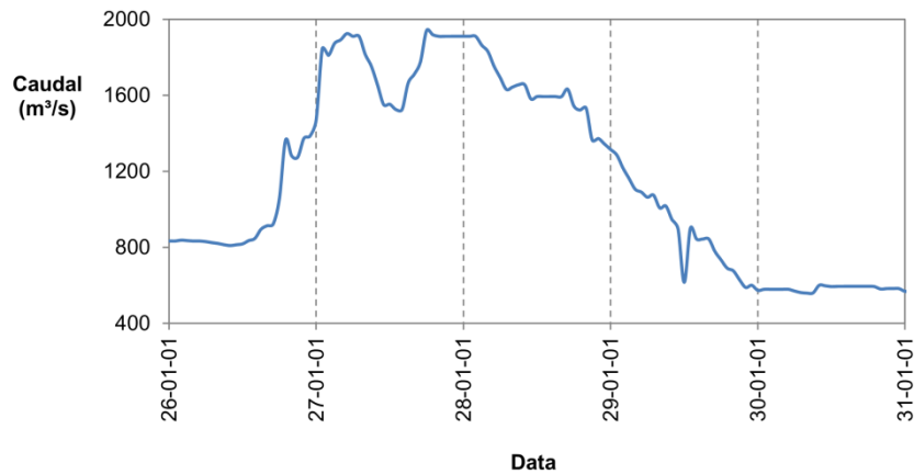
Figura 4 - Caudal afluente ao Açude-Ponte de Coimbra entre 26 e 31 de janeiro de 2001.
