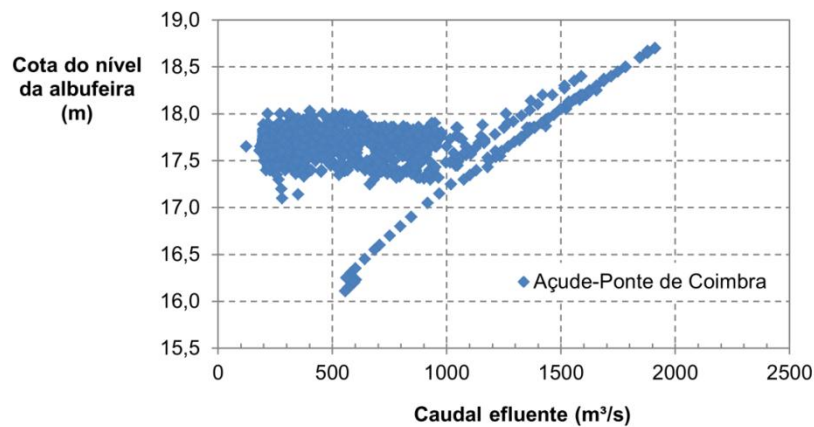
Figura 5 - Relação entre cotas do nível na albufeira do Açude-Ponte de Coimbra e caudais descarregados no período de 1 de dezembro de 2000 a 31 de janeiro de 2001.
