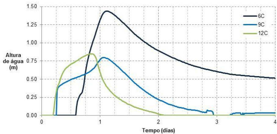
Figura 10 - Alturas de água nos pontos 12C, 9C e 6C para o cenário III.
