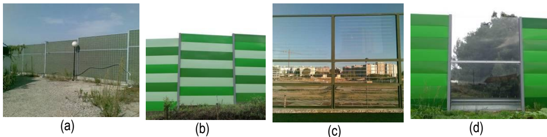
Figura 1 – Fotografias de barreiras acústicas apresentadas no questionário, (a) Fotografia 1 (barreira verde); (b) Fotografia 2 (barreira em painéis metálicos); (c) Fotografia 3 (barreira em acrílico) e (d) Fotografia 4 (barreira mista)
