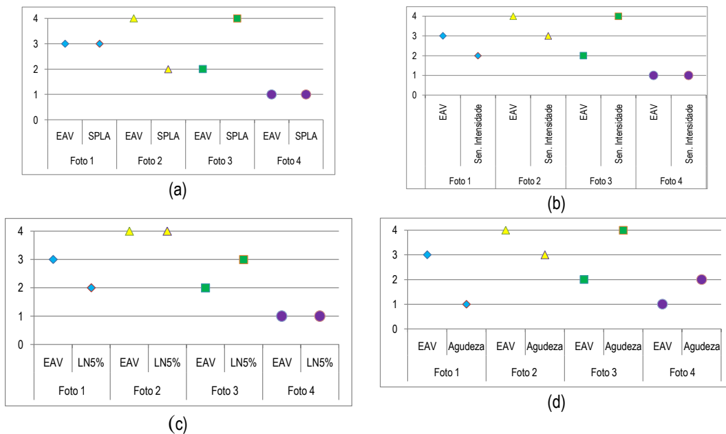
Figura 7 – Ordenação para a eficácia audiovisual (EAV) na apresentação simultânea da fotografia e registo áudio associado por detrás da barreira acústica (escala entre a mais eficaz (1) até a menos eficaz (4)), e da agudeza, de cada registo áudio, ordenado desde o menor valor (1) até ao maior valor (4), e do nível sonoro, ponderada A (a), sensação de intensidade auditiva (b), nível percentil de 5% (c), e agudeza (d) de cada registo áudio, ordenado desde o menor valor (1) até ao maior valor (4)
