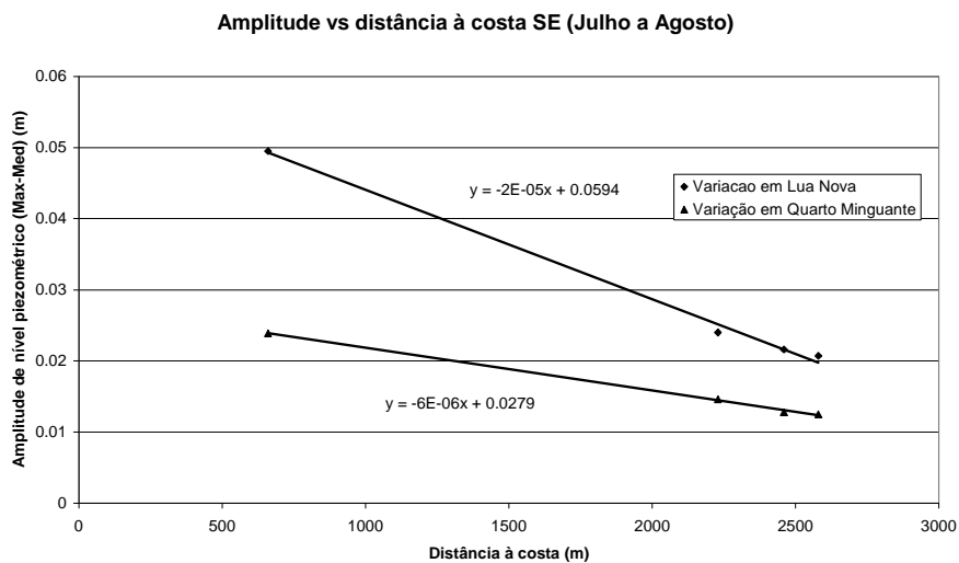
Fig. 6 - Variação do nível piezométrico (Max-Med) versus distância à costa SE (período de registo de Julho a Agosto)
