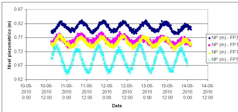
Fig. 3 - Amplitude de maré registada nos diferentes piezómetros (exemplo do período de 10-08-2010 a 14-08-2010 - Lua Nova)
