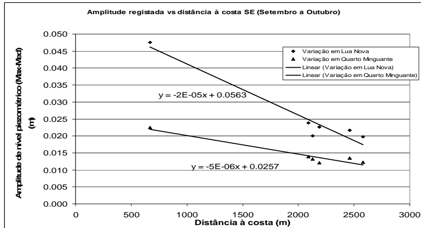
Fig. 7 - Variação do nível piezométrico (Max-Med) versus distância à costa SE (período de registo de Setembro a Outubro)
