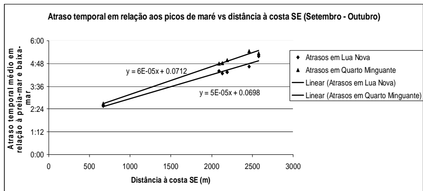
Fig. 5 - Atraso temporal médio em relação à baixa-mar ou preia-mar versus distância à costa SE (período de registo de Setembro a Outubro)
