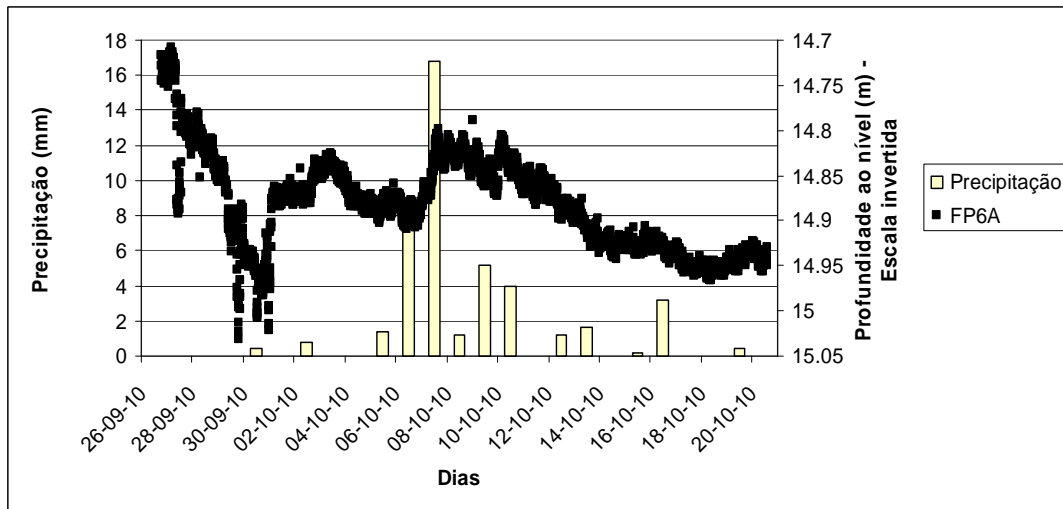
Fig. 2 – Profundidade ao nível registada no piezómetro FP6A e precipitação diária registada na Praia da Vitória
