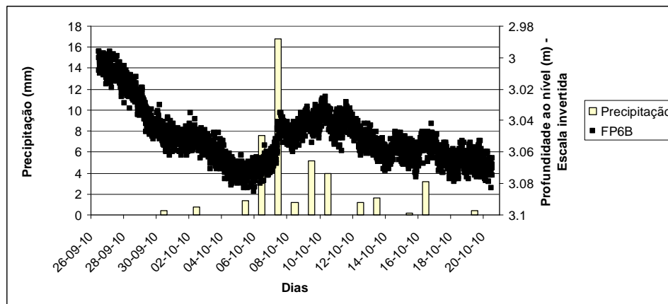
Fig. 1 – Profundidade ao nível registrada no piezómetro FP6B e precipitação diária registrada na Praia da Vitória
