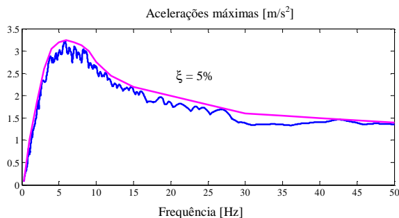
Fig. 20 – Espectro de resposta envolvente utilizado no estudo do comportamento sísmico da torre.
