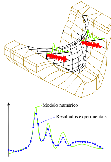
Fig. 1 – Utilização integrada de resultados de observação do comportamento dinâmico e de resultados numéricos.
