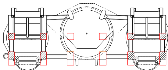
Fig. 7 – Torre das tomadas de água: vista em planta. Simplificações adoptadas na definição das secções dos pilares no modelo numérico (zona superior da torre).
