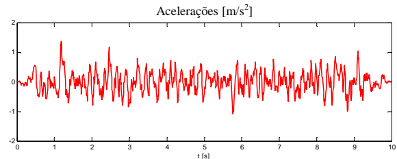
Fig. 18 – Acelerograma sísmico considerado no estudo do comportamento sísmico da torre.
