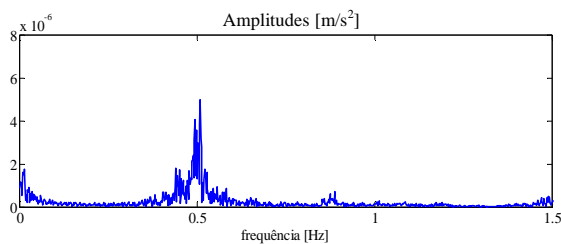
Fig. 17 – Espectro de amplitudes correspondente ao acelerograma medido na direcção margem esquerda-direita.
