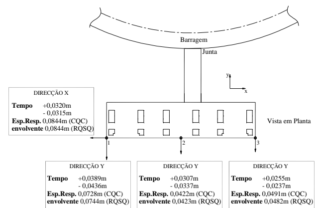
Fig. 21 – Deslocamentos sísmicos máximos em três pontos no topo da torre, utilizando o modelo 3D em SAP 2000. Comparação da análise no domínio do tempo e com base no espectro de resposta envolvente (RQSQ e CQC).
