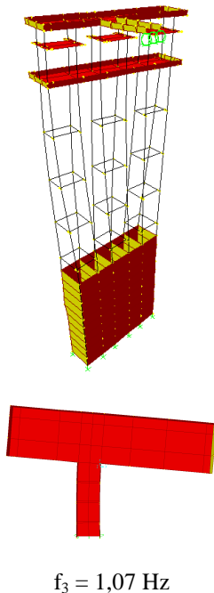
Fig. 9 – 3º modo de vibração e respectiva frequência natural obtida com o modelo 3D em SAP 2000.
