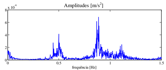
Fig. 14 – Espectro de amplitudes correspondente ao acelerograma medido na direcção montante-jusante.
