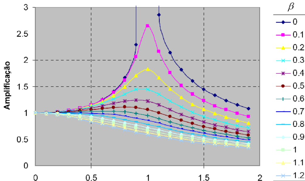
Fig. 7-Amplificação dinâmica versus factor velocidade ( \alpha ) para diversos valores do factor de amortecimento ( \beta )
