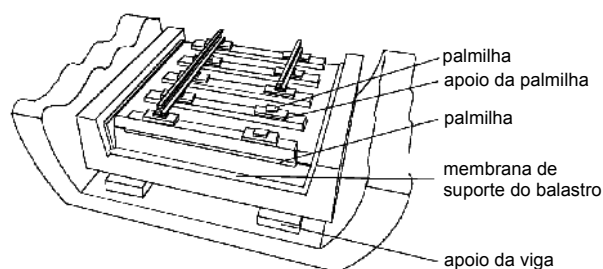
Fig. 11 - Sistema massa-mola para controlo de vibrações
