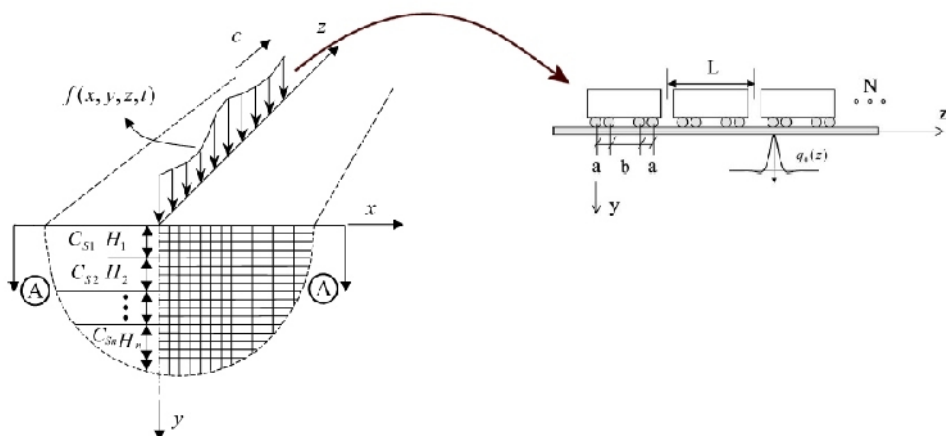
Fig. 3-Representação esquemática da geometria do problema e do sistema de cargas (Yang et al., 2003)
