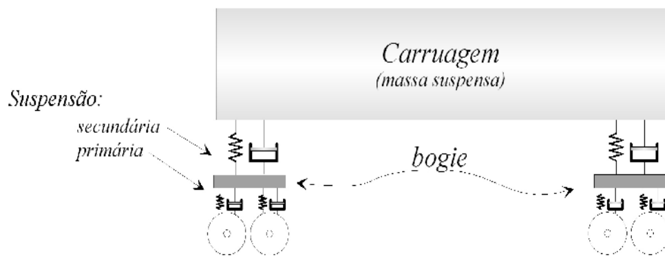
Fig. 1- Modelo analógico de carruagem com rodados, bogies e suspensões
