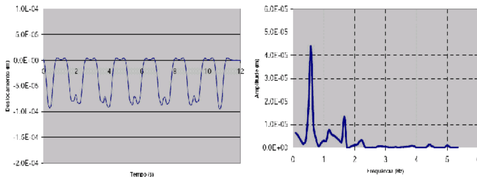
Fig. 9-Resposta da viga para o comboio alfa pendular a circular a 50 km/h (modelo de Winkler)
