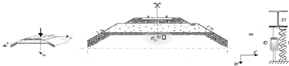
Fig. 4-Modelo de um aterro ferroviário e respectivo modelo de viga de Winkler (adaptado de Hall, 2000)
