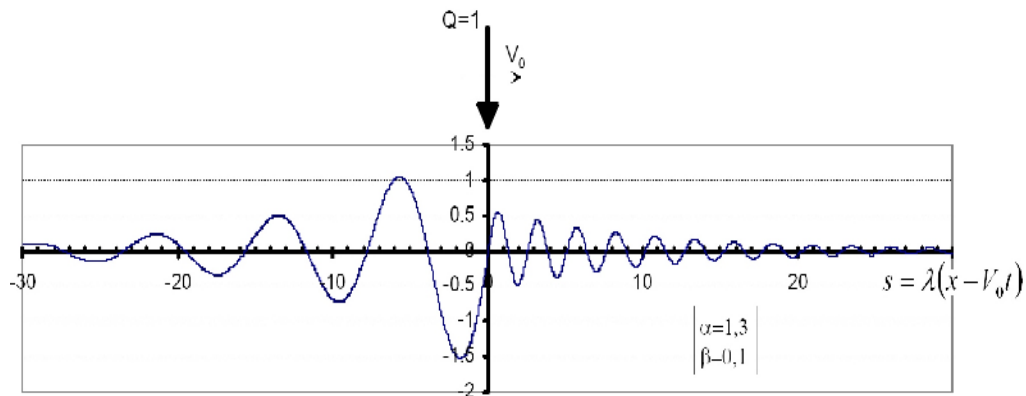
Fig. 5-Propagação das vibrações no modelo da viga de Winkler e efeito de Doppler
