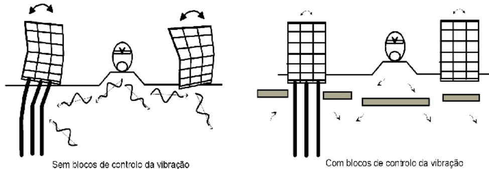
Fig. 10-Funcionamento dos blocos de controle de vibração (adaptado de Takemiya et al., http://www.aisawa.co.jp )
