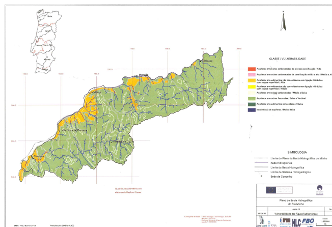
Figura 4 – Mapeamento obtido pelo método EPNA da vulnerabilidade à poluição das águas subterrâneas da bacia hidrográfica do rio Minho, em Portugal, desenvolvida por Novo et al. (2000).
