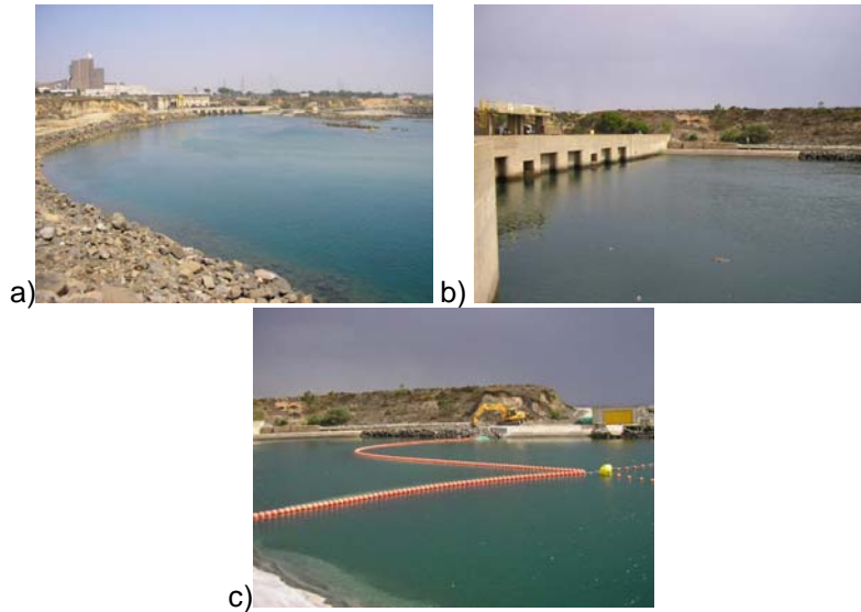
Figura 2: a) Interior da bacia de adução; b) Localização das bombas; c) Redes.
