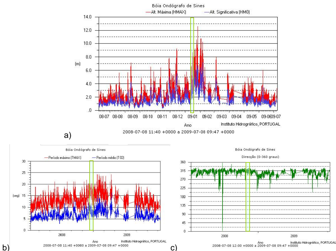
Figura 6: Valores temporais de: a) altura de onda máxima e significativa; b) Período máximo e período médio; c) Direcção, no período de 15-07-2008 a 15-07-2009.
