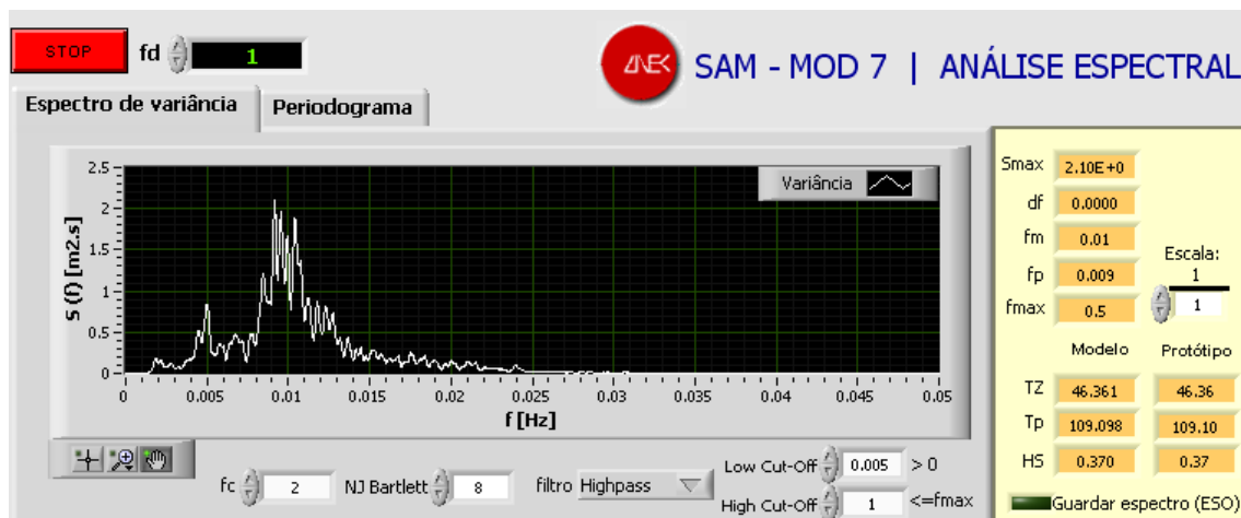
Figura 4: Análise espectral dos dados medidos no período de 18 de Janeiro às 22h a 19 de Janeiro às 22h.
