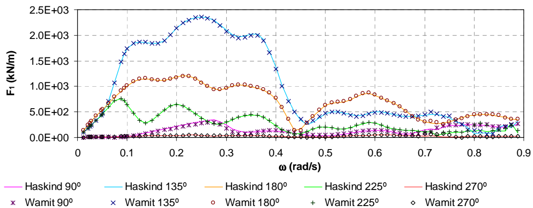
Fig. 6. Evolução, com a frequência e a direcção de propagação da onda, da força segundo o avanço. Comparação dos resultados do problema de difracção com os obtidos da implementação das relações de Haskind. Ondas incidentes em navio a 15 m de parede vertical em zona com 18 m de profundidade.
