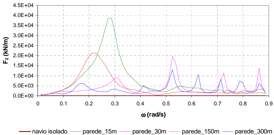
Fig. 4. Evolução, com a frequência e a distância à parede, da força segundo o abatimento. Resultados do problema de difração. Ondas de vante incidentes em navio próximo de parede vertical em zona com 18 m de profundidade.
