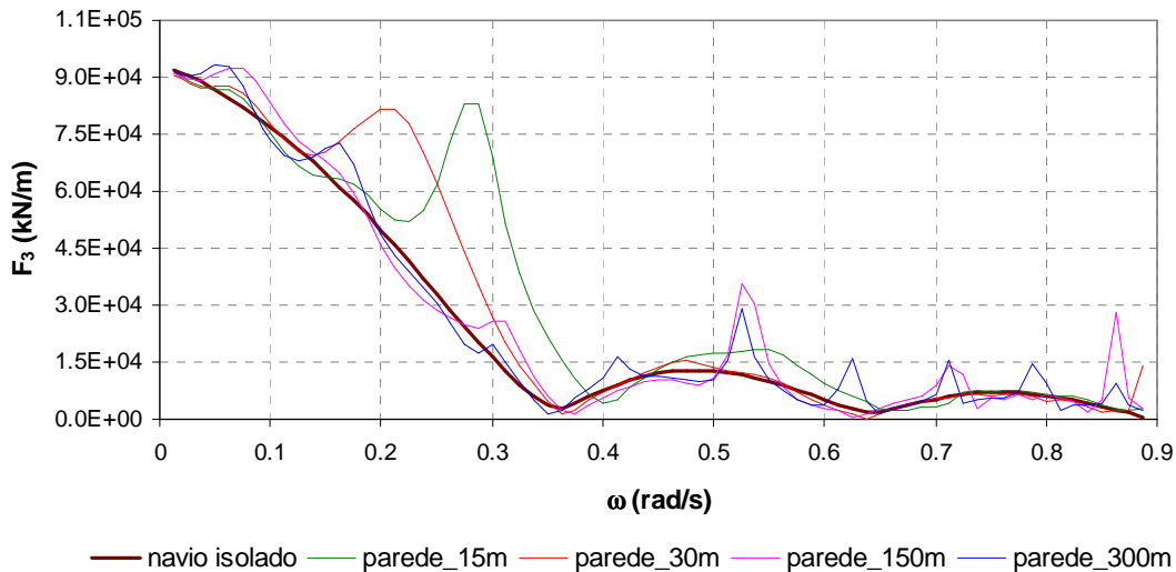
Fig. 5. Evolução, com a frequência e a distância à parede, da força segundo a arfagem. Resultados do problema de difracção. Ondas de vante incidentes em navio próximo de parede vertical em zona com 18 m de profundidade.
