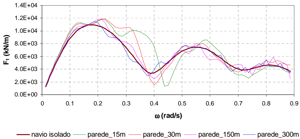
Fig. 3. Evolução, com a frequência e a distância à parede, da força segundo o avanço. Resultados do problema de difração. Ondas de vante incidentes em navio próximo de parede vertical em zona com 18 m de profundidade.
