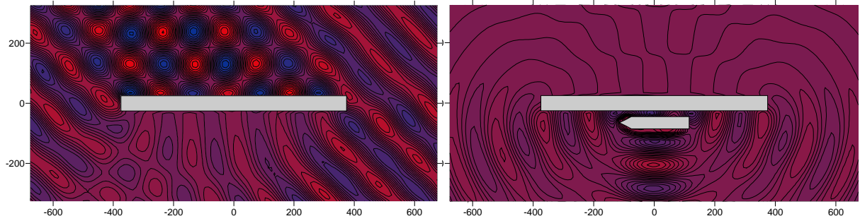
Fig. 2. Elevação da superfície para frequência de 0.5125 rad/s. a) ondas incidentes na parede isolada fazendo um ângulo de 225° com o eixo x do sistema de eixos global; b) oscilação forçada do navio segundo o modo de arfagem
