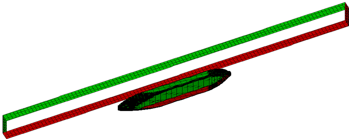
Fig. 1. Esquema da painelização do navio e da parede simulados.
