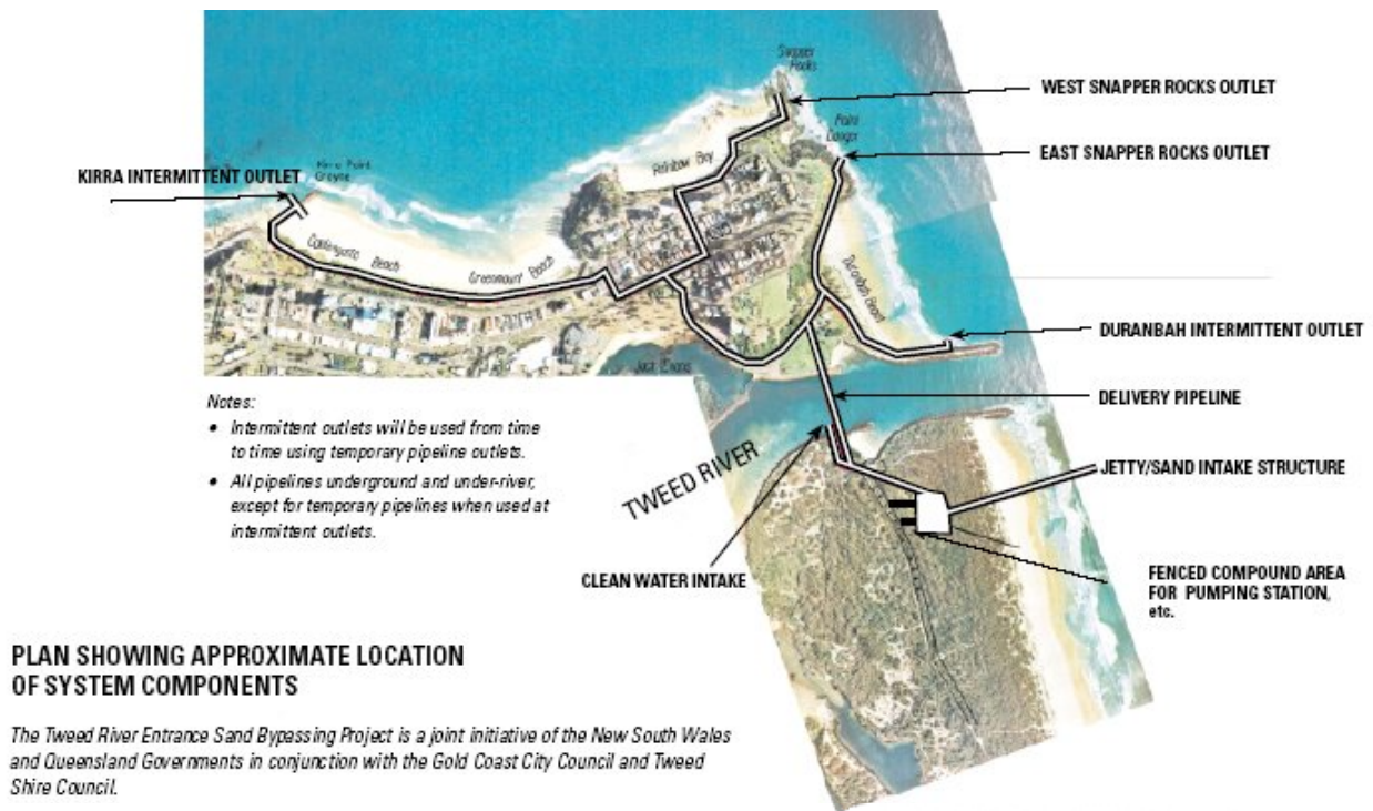
Figura 9 – Sistema de transposição de areias na embocadura do rio Tweed, Austrália (fonte: www.epa.qld.gov.au/sandbypass ). Tweed River Entrance sand bypassing system, Austrália (source: www.epa.qld.gov.au/sandbypass ).
