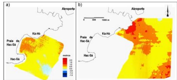
Figura 13 – Evolução morfológica do fundo marítimo: a) entre 1985 e 2002; b) entre 1985 e 2001. Morphological evolution: a) between 1985 and 2002; b) between 1985 and 2001.
