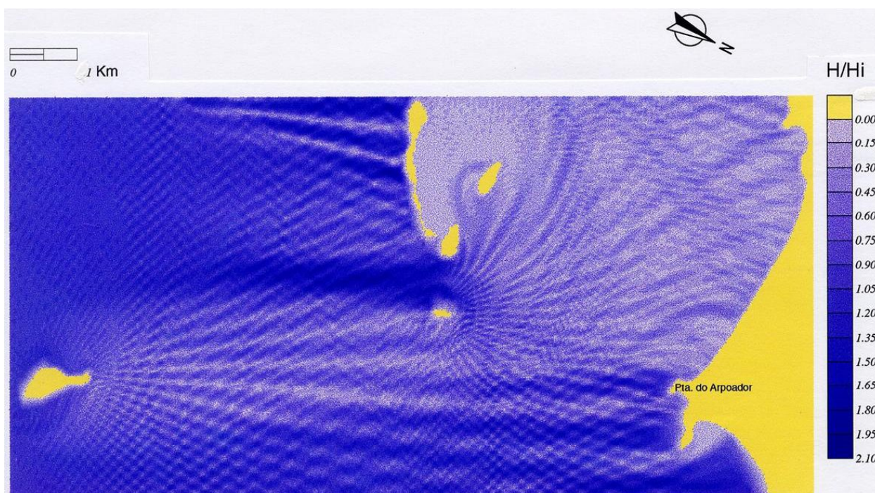
Figura 16 – Propagação da agitação marítima desde o largo até às praias de Leblon, Ipanema e Arpoador. Exemplo de resultados obtidos com um modelo matemático. Wave propagation from the ocean to the beaches of Leblon, Ipanema and Arpoador. Example of results from a mathematical model.
