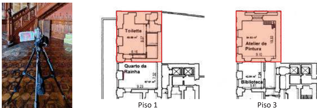
Figura 9 – Locais de medição e equipamento de termografia de infravermelhos (TIV)
