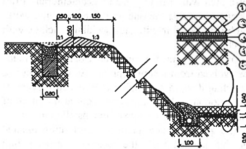
Fig. 4. Liner system: (1) subgrade; (2) geotextile; (3) geomembrane; (4) geotextile; (5) sand.
