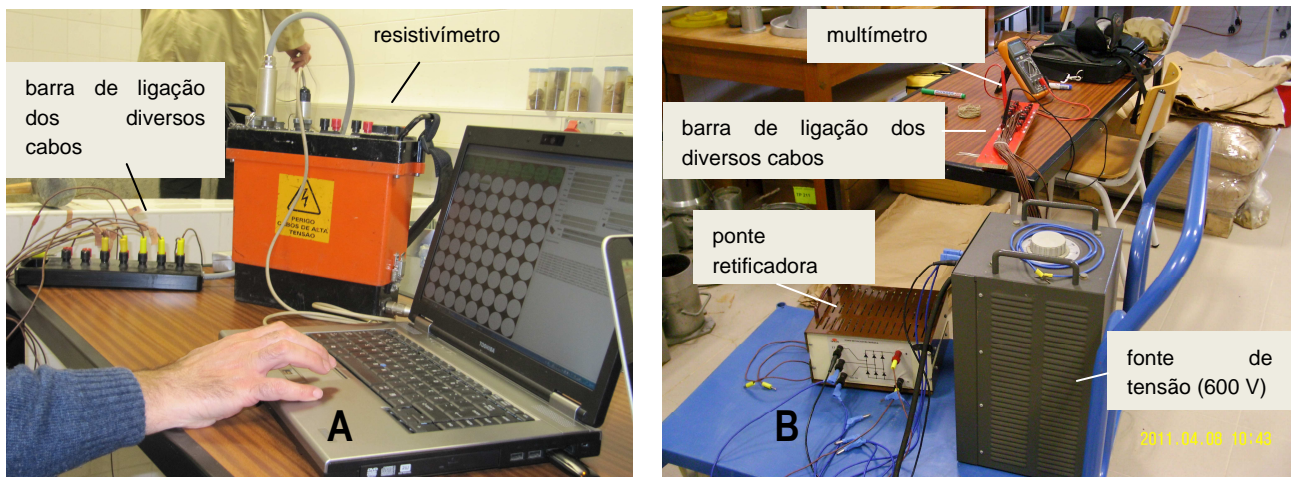
Figura 6 - Equipamento de injeção e medição utilizado na célula experimental do ISEL. A – resistívmetro; B – fonte de tensão de 600V.
