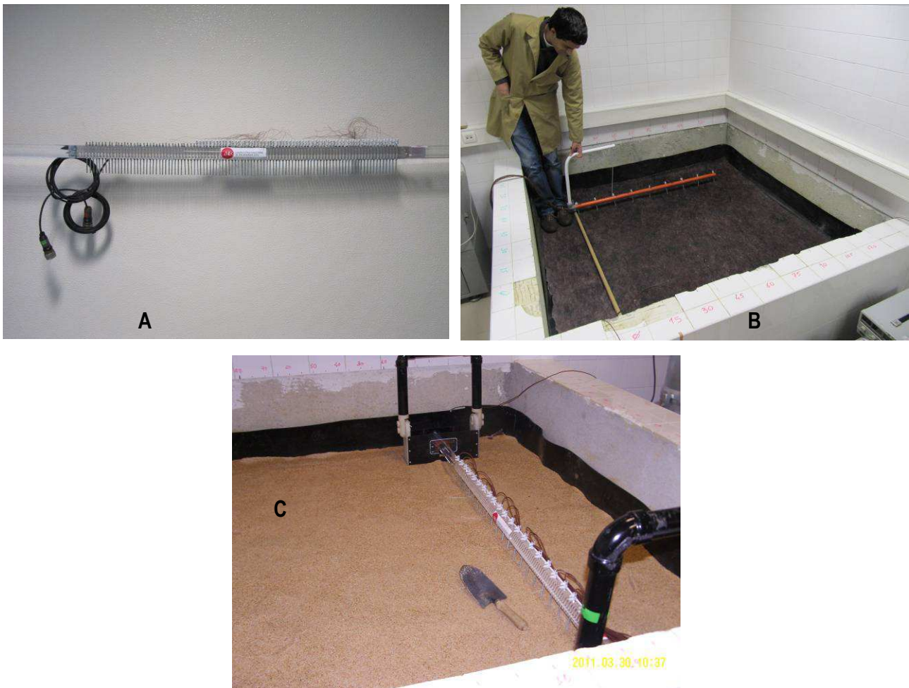
Figura 5 – Protótipos de pequena escala. A – Espaçamento entre elérodos de 1 cm; B – Espaçamento entre elérodos de 15 cm; C – Espaçamento entre elérodos de 5 cm.
