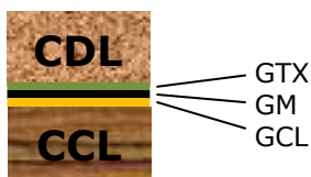
Figura 1 – Sistema de impermeabilização de fundo dos aterros de resíduos
