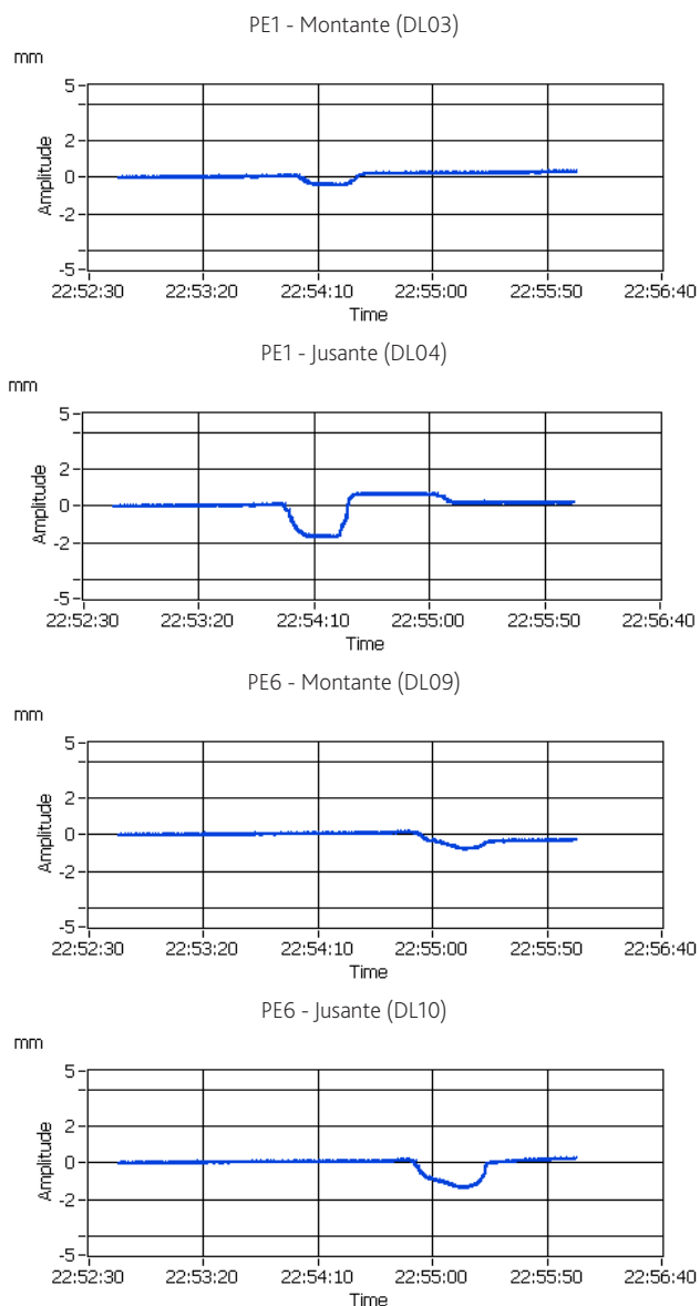
Figura 14 Deformação dos LUD durante a passagem do comboio do serviço regular
