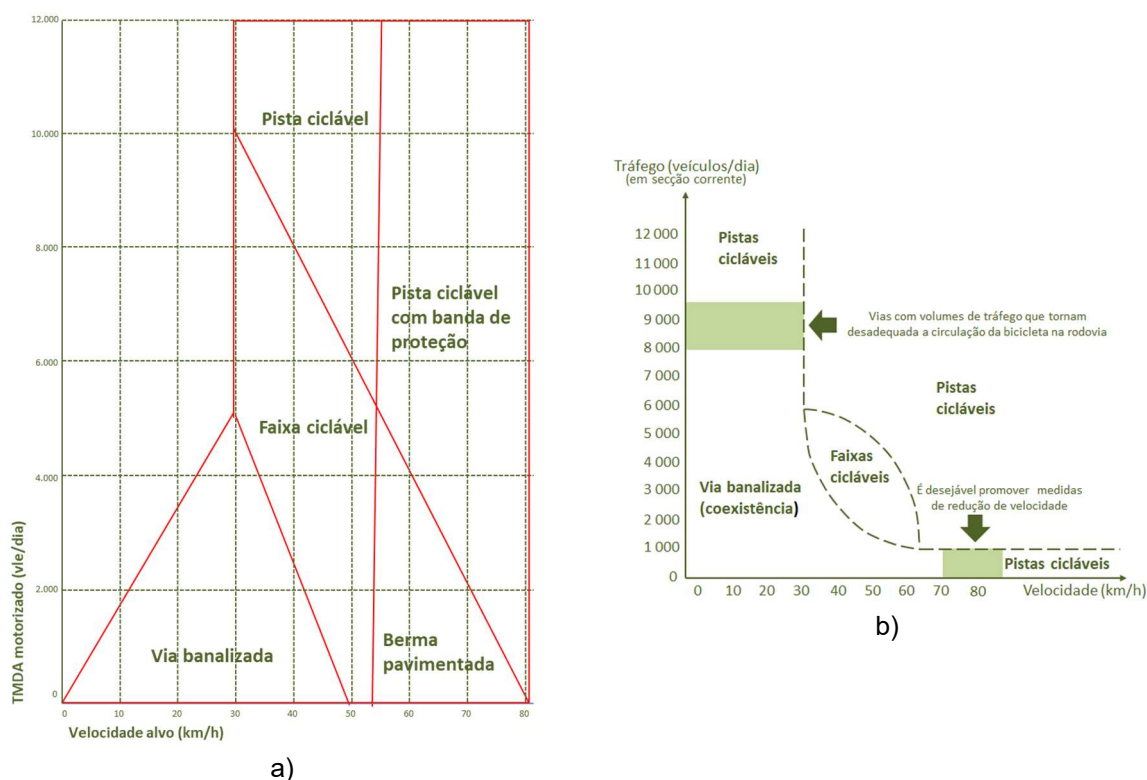
Figura 3.1 – Seleção do tipo de percurso ciclável (adaptado de Veidirektoratet, 2000 e CERTU, 1998)
