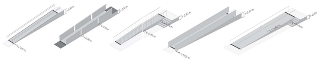
Figura 2.15 – Prática de rampas recomendada para segurança dos utilizadores mais vulneráveis (SNRIPD, 2006)
