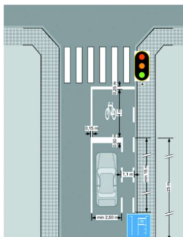
Figura 3.16 – Interseção com sinalização luminosa e faixa ciclável (DGT, 2009, referido em IMTT, I.P., 2011b).
