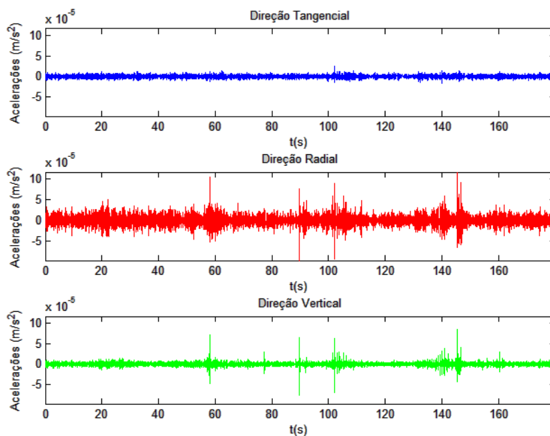
Fig. 6 - Posição do acelerómetro triaxial (Nanometrics) e respetivas séries temporais recolhidas no ensaio de vibração ambiente para a situação de albufeira vazia (Ensaio 1), para as direções tangencial, radial e vertical
