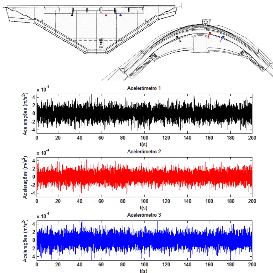
Fig. 7 - Posição dos acelerómetros uniaxiais (Kinematics) e respectivas séries temporais recolhidas no ensaio de vibração ambiente para a situação de albufera cheia (Ensaio 2)
