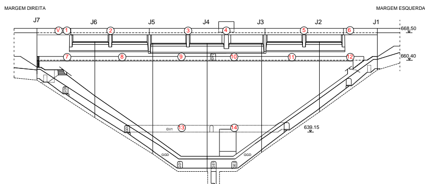
Fig. 5 - Plano de colocação da aparelhagem utilizada durante o ensaio de vibração forçada
