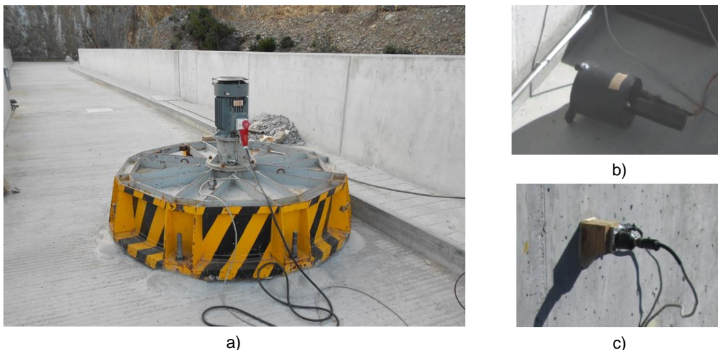
Fig. 4 - Pormenores de colocação: a) vibrador de massa excêntrica, b) transdutor de velocidade e c) acelerómetro.
