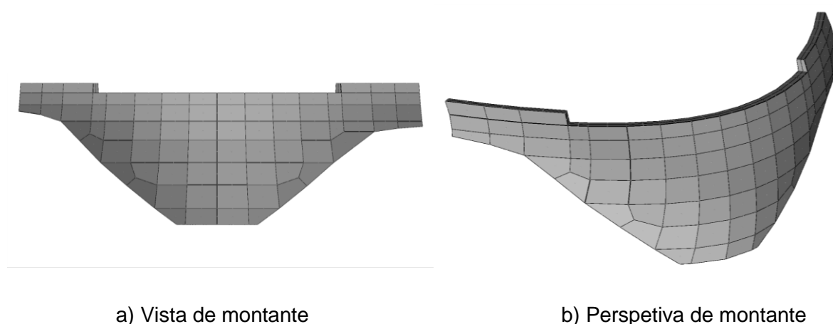
Fig. 8 - Malha de elementos finitos do modelo numérico do corpo da barragem
