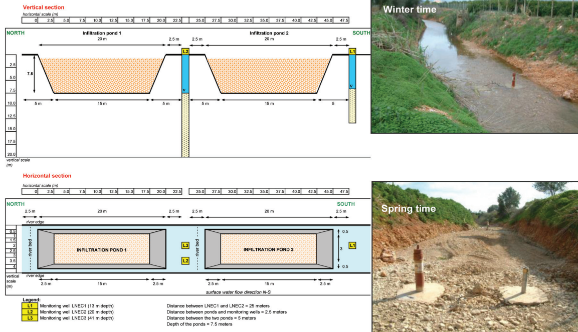
Fig. 4 - Design configuration of the two infiltration basins in the river bed of Rio Seco (at Carreiros), winter time and spring time photos. Fig. 4 - Schema dei due bacini di infiltrazione nel letto del Rio Seco (a Carreiros), nelle foto il periodo invernale e primaverile.
