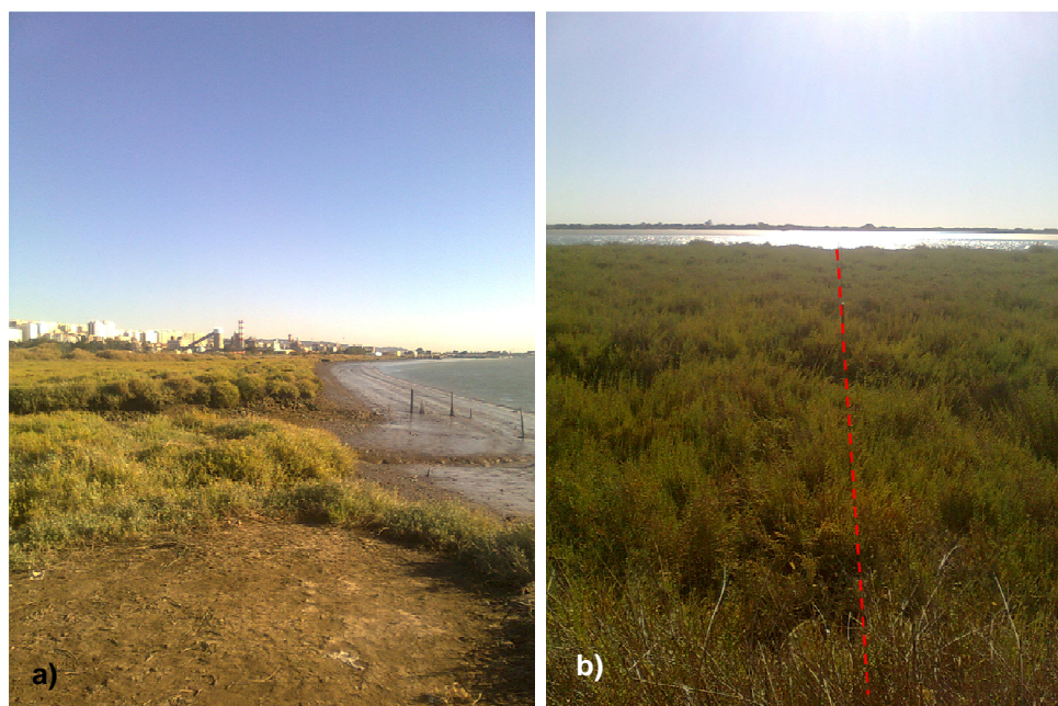
Fig. 3 – a) Vista geral do sapal 1 junto ao Tejo e raso de maré adjacente, vista para NE; b) alinhamento de um dos perfis levantados, vista para SE (ponto Sapal 1 na Fig. 1)
