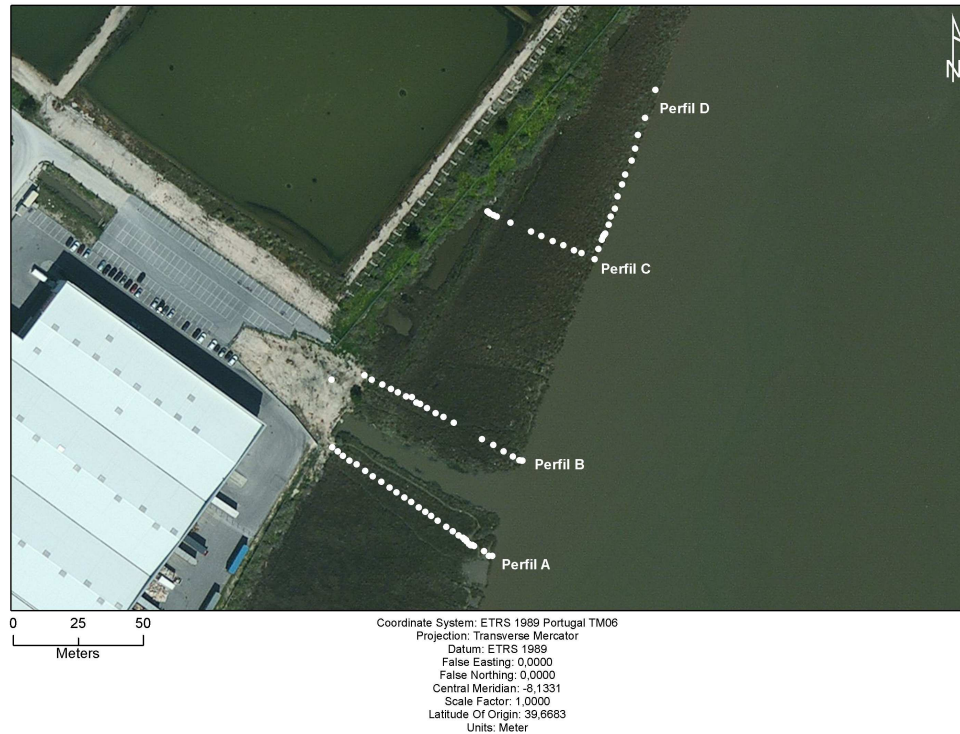
Fig.2 – Perfis topográficos levantados no sapal 1
