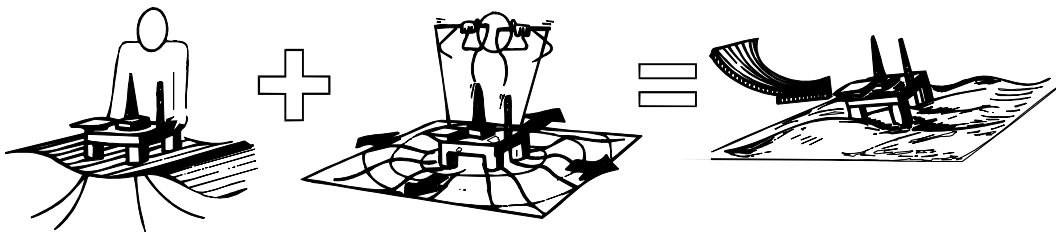
Figura 2. Decomposição da interacção de um corpo flutuante com as ondas nos problemas de difracção e de radiação, adaptado de Faltinsen (1990).
