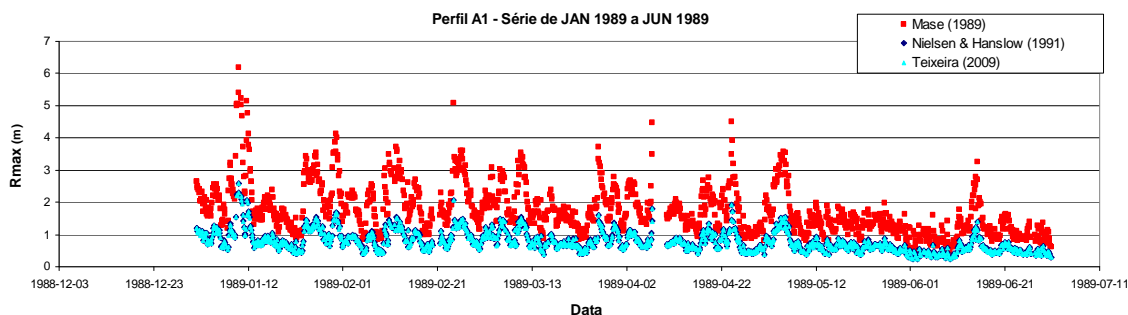
Figura 6 – Valores do máximo espraioamento, R_{max} , obtidos no Perfil A1 para o período entre Janeiro e Junho de 1989, através das fórmulas de MASE (1989), NIELSEN & HANSLOW (1991) e TEIXEIRA (2009) para as condições de agitação marítima ao largo.
