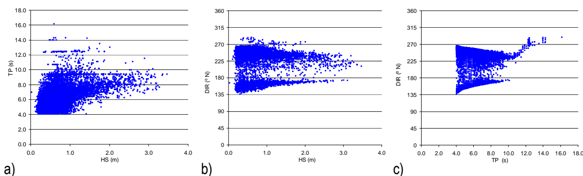
Figura 5 – Relações HS-TP, HS-DIR e TP-DIR no Ponto 9 para os anos de 1986 a 1995.
