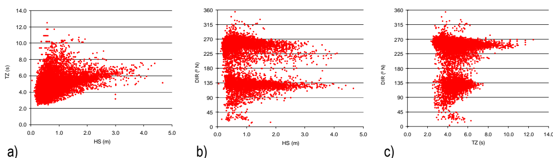
Figura 3 – Relações HS-TZ, HS-DIR e TZ-DIR na bóia-ondógrafo de Faro para os anos de 1986 a 1995.
