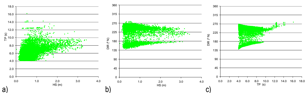
Figura 4 – Relações HS-TP, HS-DIR e TP-DIR no Ponto 6 para os anos de 1986 a 1995.
