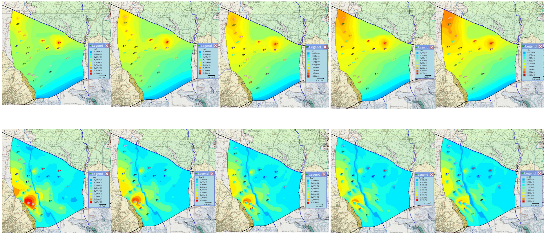
Injecção 25 noras
