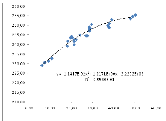
Figura 1: relação entre os parâmetros OIT estático e dinâmico à temperatura de 210°C
